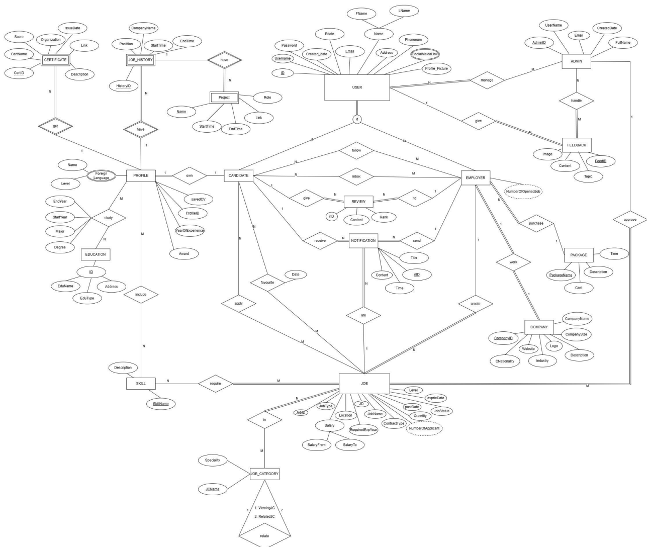
Hình 16: Sơ đồ quan hệ thực thể (ERD)
