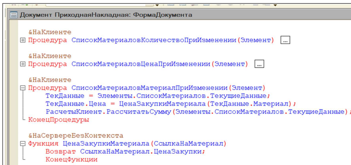
Рисунок 2 – Механизм подстановки цены
