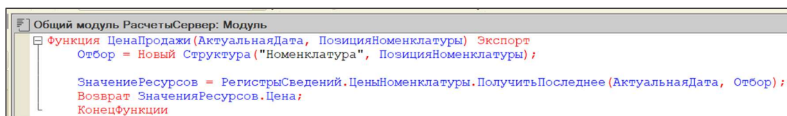
Рисунок 3 – Функция запроса актуальной цены заданного элемента
