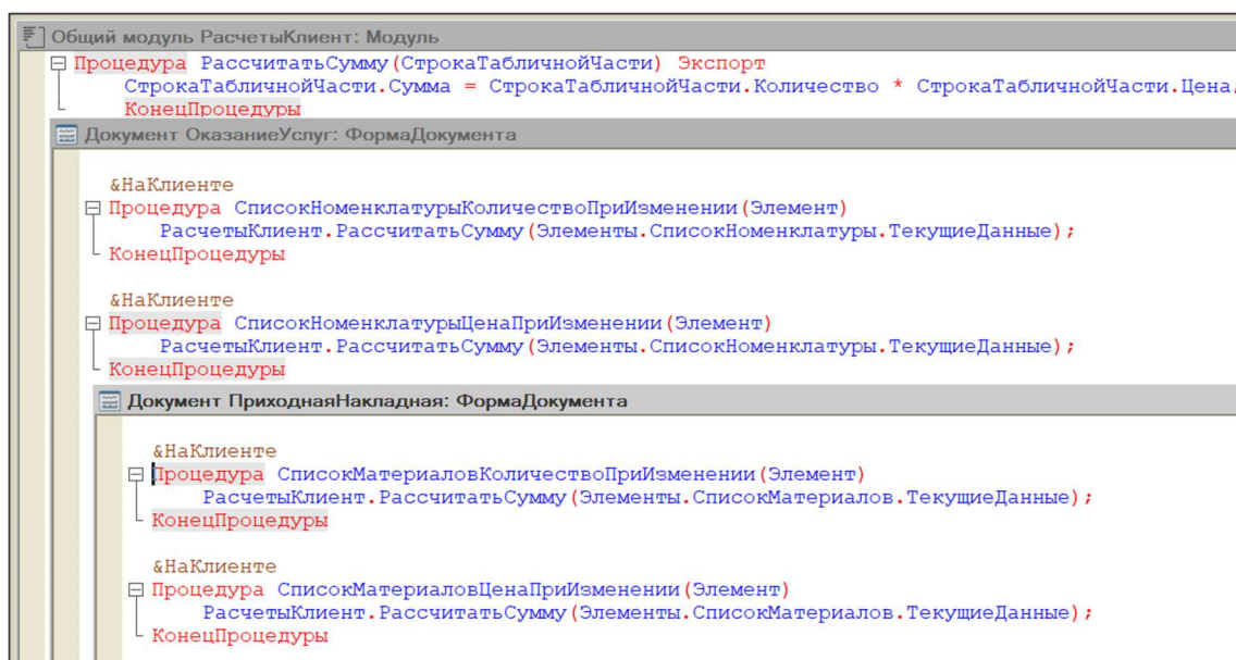
Рисунок 1 – Модули расчёта суммы
