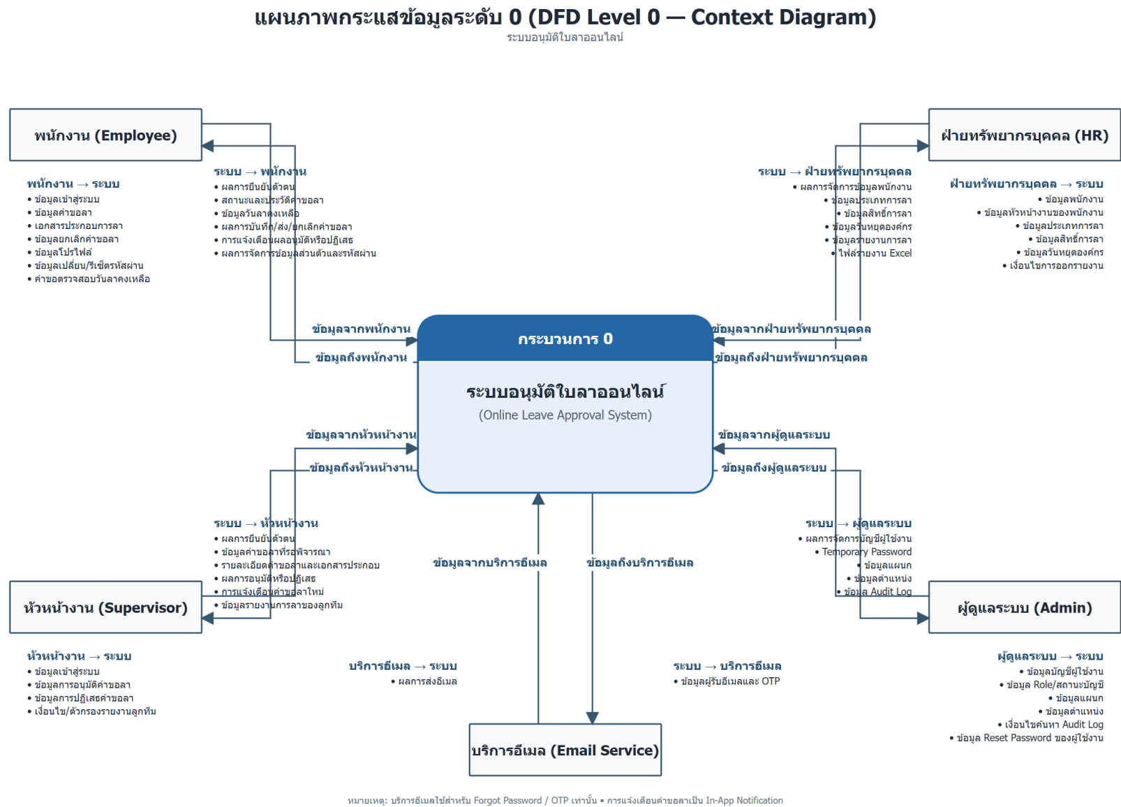
รูปที่ 2 แผนภาพกระแสข้อมูลระดับ 0 (DFD Level 0 — Context Diagram)
