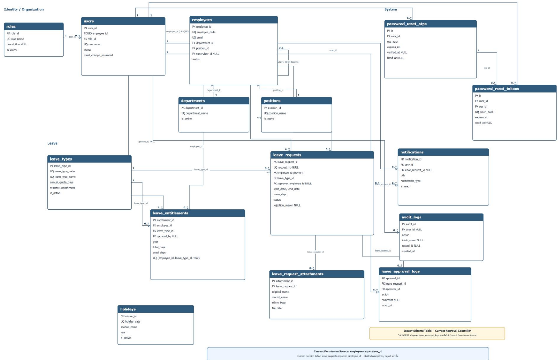
รูปที่ 5 แผนภาพความสัมพันธ์ระหว่างข้อมูล (Entity Relationship Diagram: ERD)
