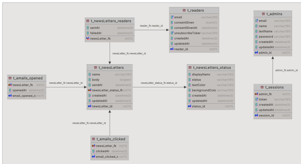
Figure 21. Schéma de la base de données
