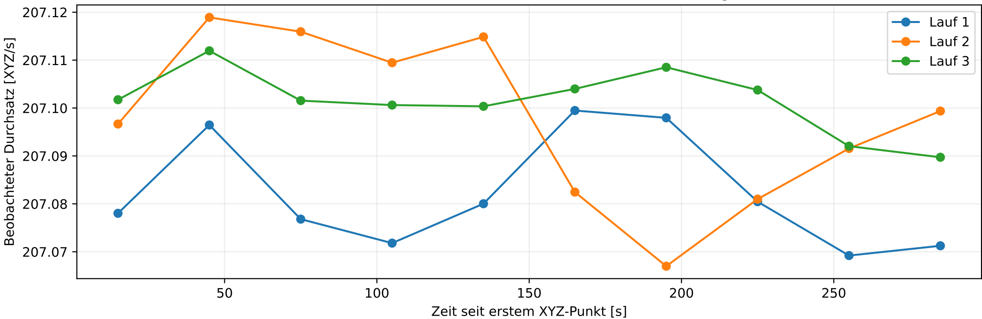
Durchsatz in 30-s-Abschnitten; nominelle Sensoreinstellung: 200 Hz
