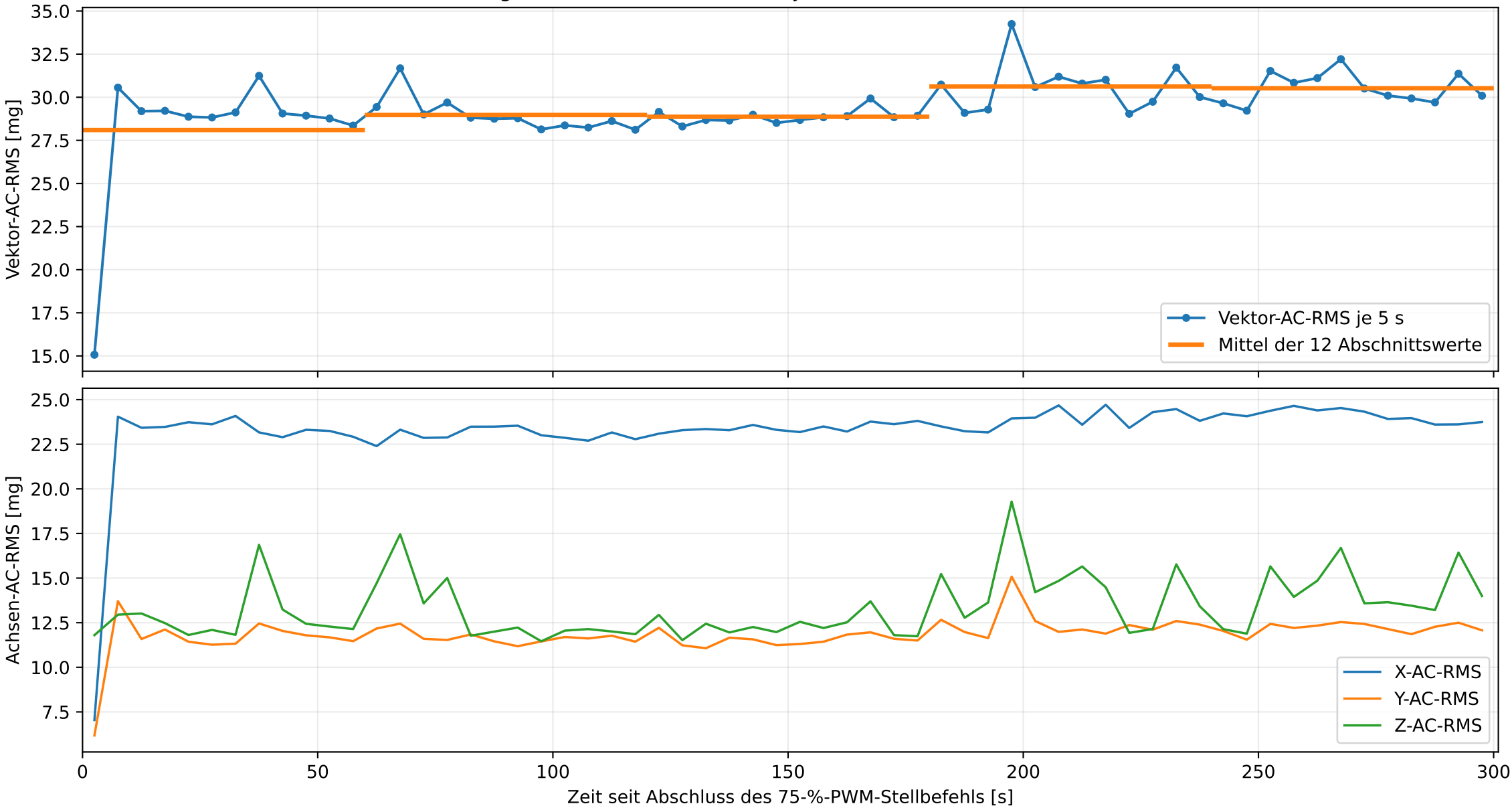
75 % PWM bei 25 kHz: einmaliger fünfminütiger Einlaufversuch Erster XYZ-Punkt 29.5 ms nach Befehlsabschluss; nominell 200 Hz Eigene Achsenmittelwerte in jedem 5-s-Abschnitt entfernt
