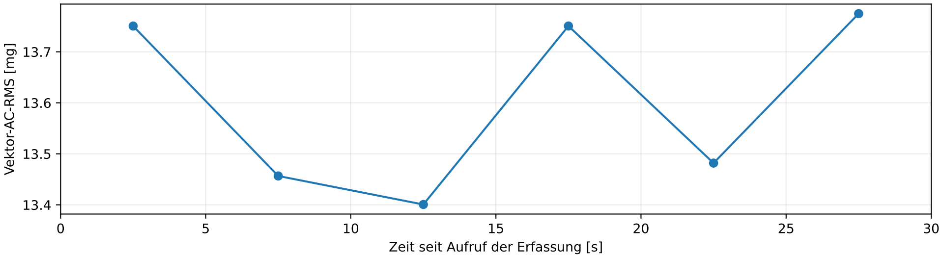
Aufrechte Aufstellung: bestätigter Stillstand, 0 % PWM Stillstandsreferenz: eigene Achsenmittelwerte je 5-s-Fenster entfernt
