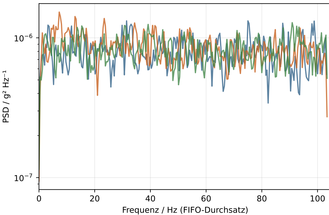
Z-Achse
