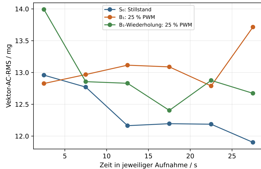
5-s-Abschnitte
