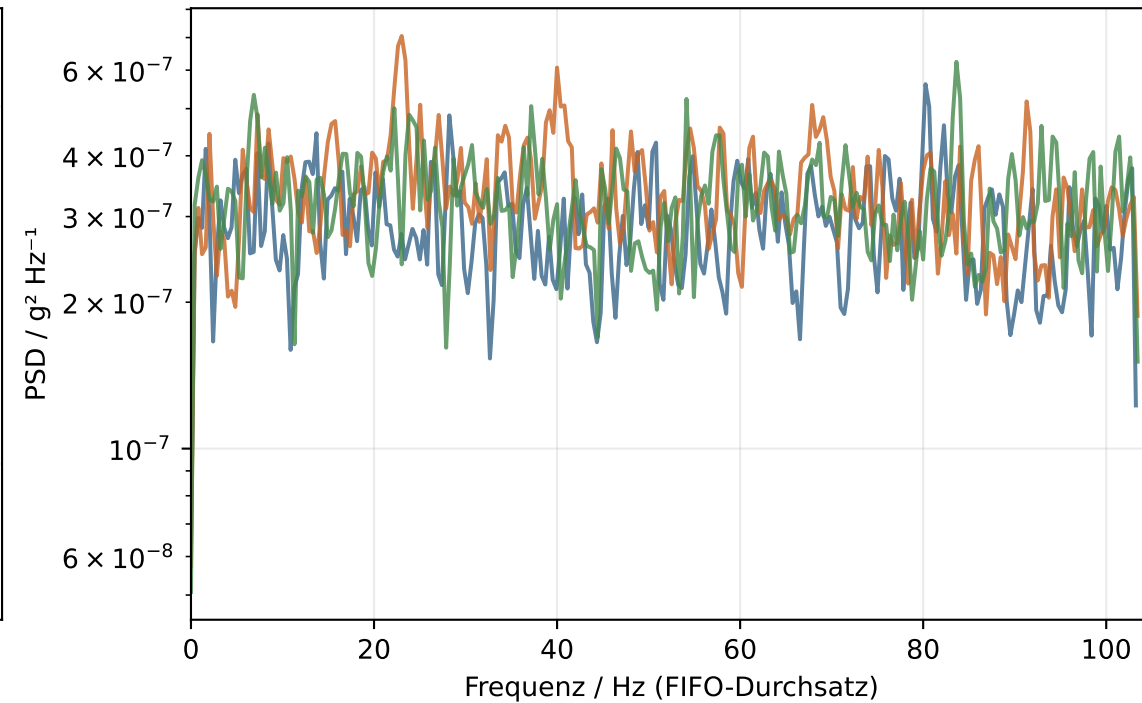
5-s-Abschnitte
