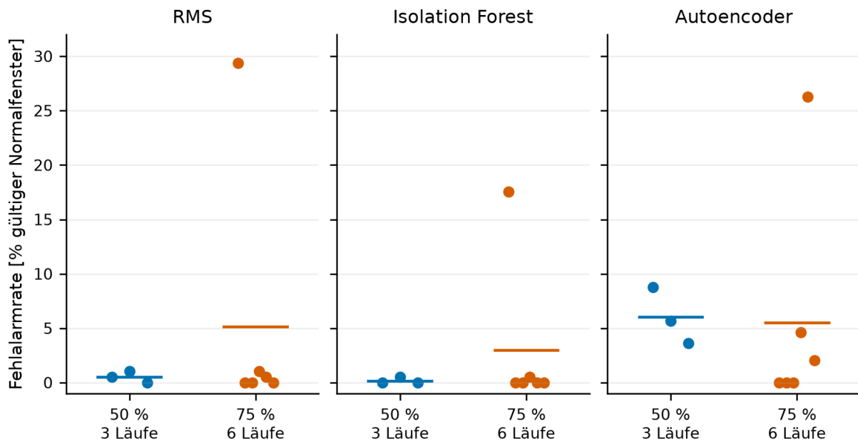
Abbildung 7-4: Fehlarmlarmraten je vollständiger Normalaufnahme und zusammengefasst bei 75 % und 50 % PWM mit demselben eingefrorenen Paket. Die Aufnahmen sind nicht zeitgleich oder randomisiert gepaart. Quelle: eigene Testauswertung.
