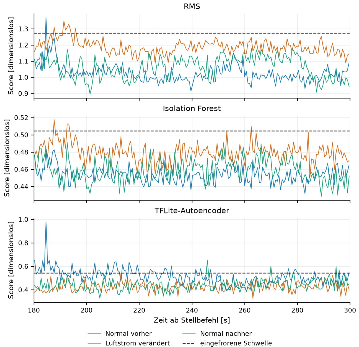
Abbildung 7-2: Eingefrorene Scores auf identischen 128er-Fenstern der unabhängigen Folge. Die gestrichelten Linien sind die vorab fixierten Schwellen. Diese Verläufe sind von den 5-s-RMS-Werten zu unterscheiden. Quelle: eigene unveränderte Testauswertung.
