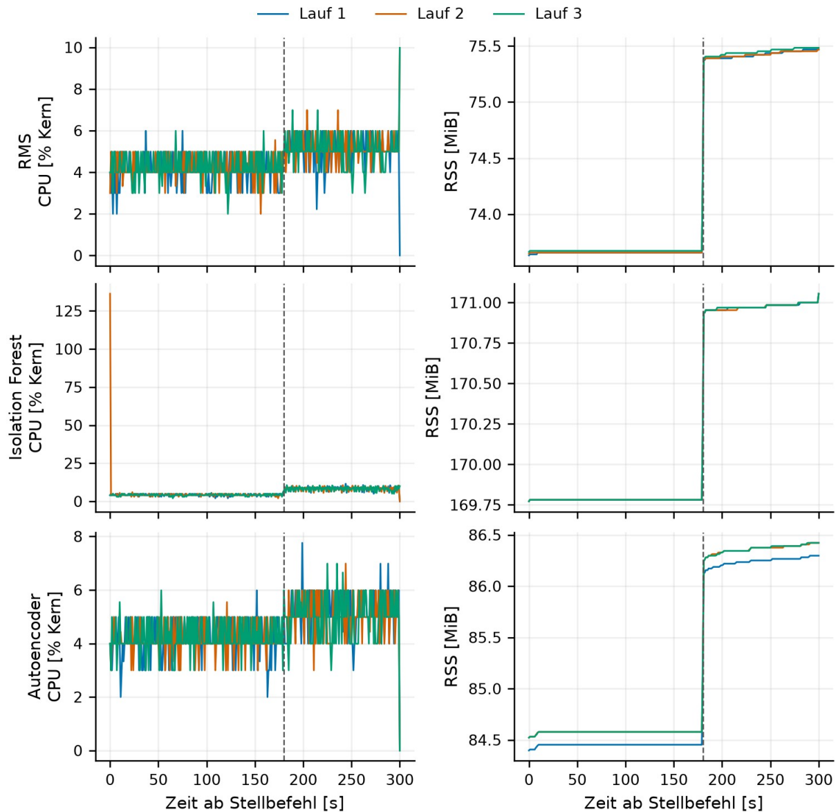
Abbildung 7-6: CPU- und RSS-Verläufe im Sensor-Livebetrieb. Zur Darstellung wurden die Ressourcenwerte in 1-s-Abschnitten gemittelt; die Kennwerte der Tabelle verwenden die ursprünglichen zeitgewichteten Messintervalle. Quelle: eigene Laufzeitmessungen.
