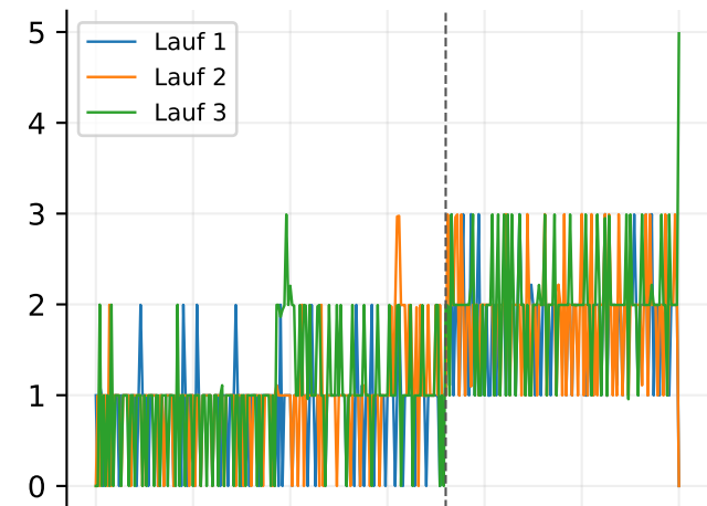
TFLite-Autoencoder
