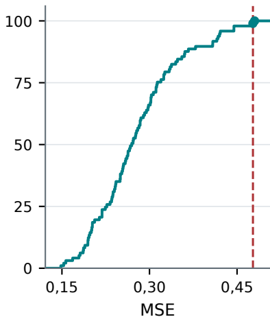
Autoencoder (Keras) Schwelle: 0,477203
