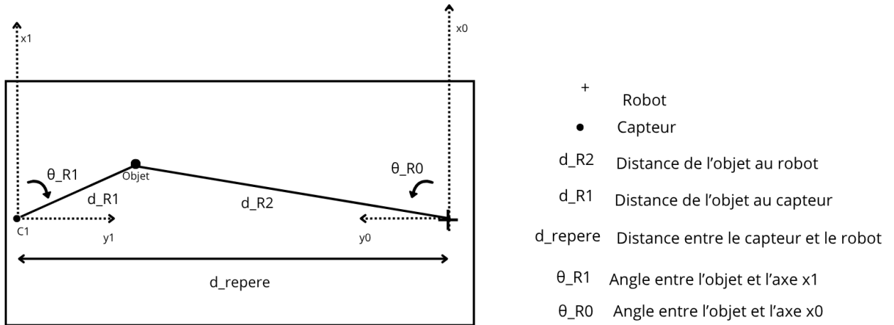
Figure 1: Schéma de la localisation angulaire avec un capteur ultrason monté sur un servo.
