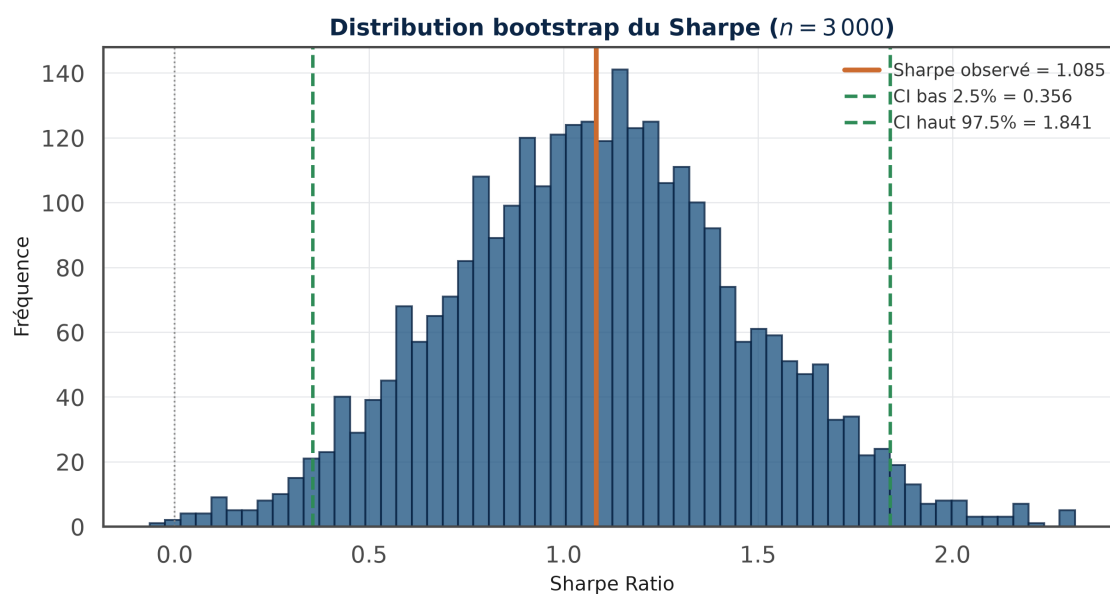
Fig. 17. Distribution bootstrap du Sharpe ratio. La ligne orange matérialise la valeur observée (1.085), les deux lignes vertes pointillées matérialisent les bornes de l'intervalle de confiance à 95 % [0.356, 1.841]. La distribution est légèrement asymétrique à droite, cohérente avec les queues épaisses des rendements FX.
