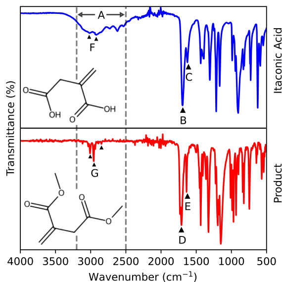
Figure 3: FT-IR spectra of reactant and product. (A) 2500-3200 \text{cm}^{-1} . (B) 1700 \text{cm}^{-1} . (C) 1630 \text{cm}^{-1} . (D) 1720 \text{cm}^{-1} . (E) 1640 \text{cm}^{-1} . (F) 2950 & 3050 \text{cm}^{-1} . (G) 2875, 2980 & 3035 \text{cm}^{-1} .
