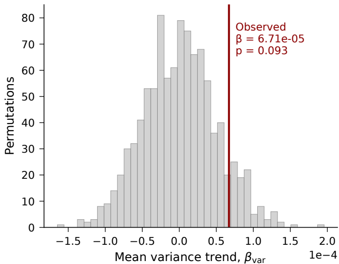
a Placebo: variance trend
