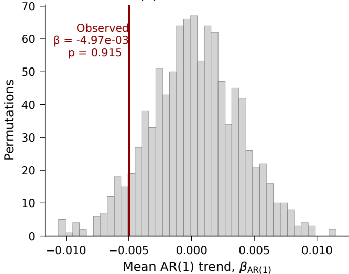
b Placebo: AR(1) trend
