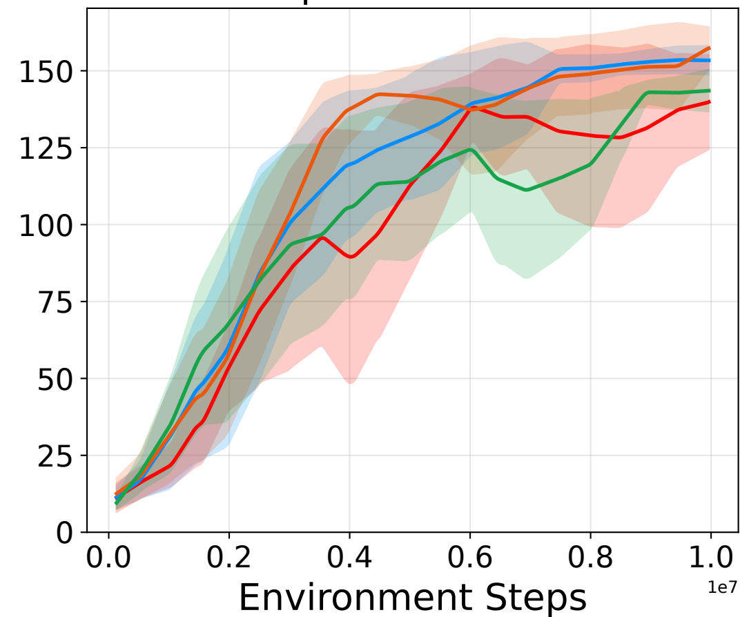
SpaceInvaders
