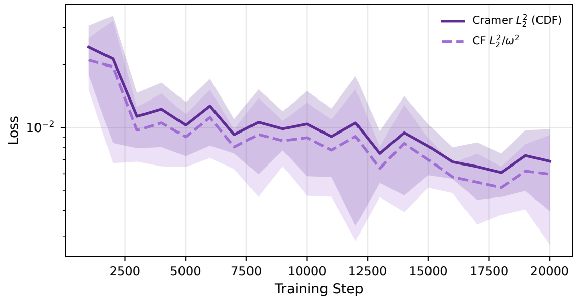
Parseval anchor
