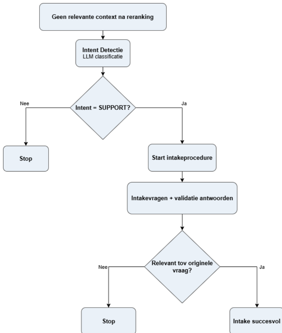
Figuur 25: Intake flow
