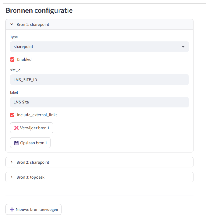
Figuur 50: Overzicht bestaande bronnen
