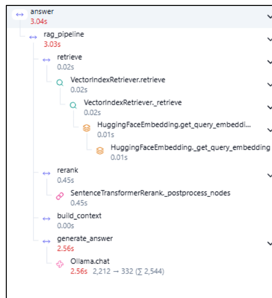
Figuur 61: Trace van volledige flow
