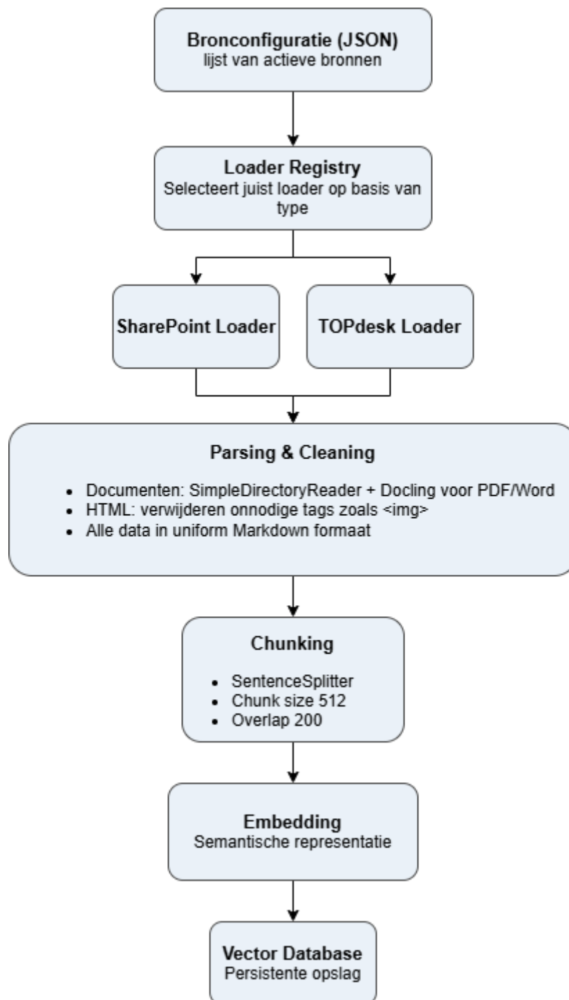
Figuur 8: Ophalen data met opslag in vector database
