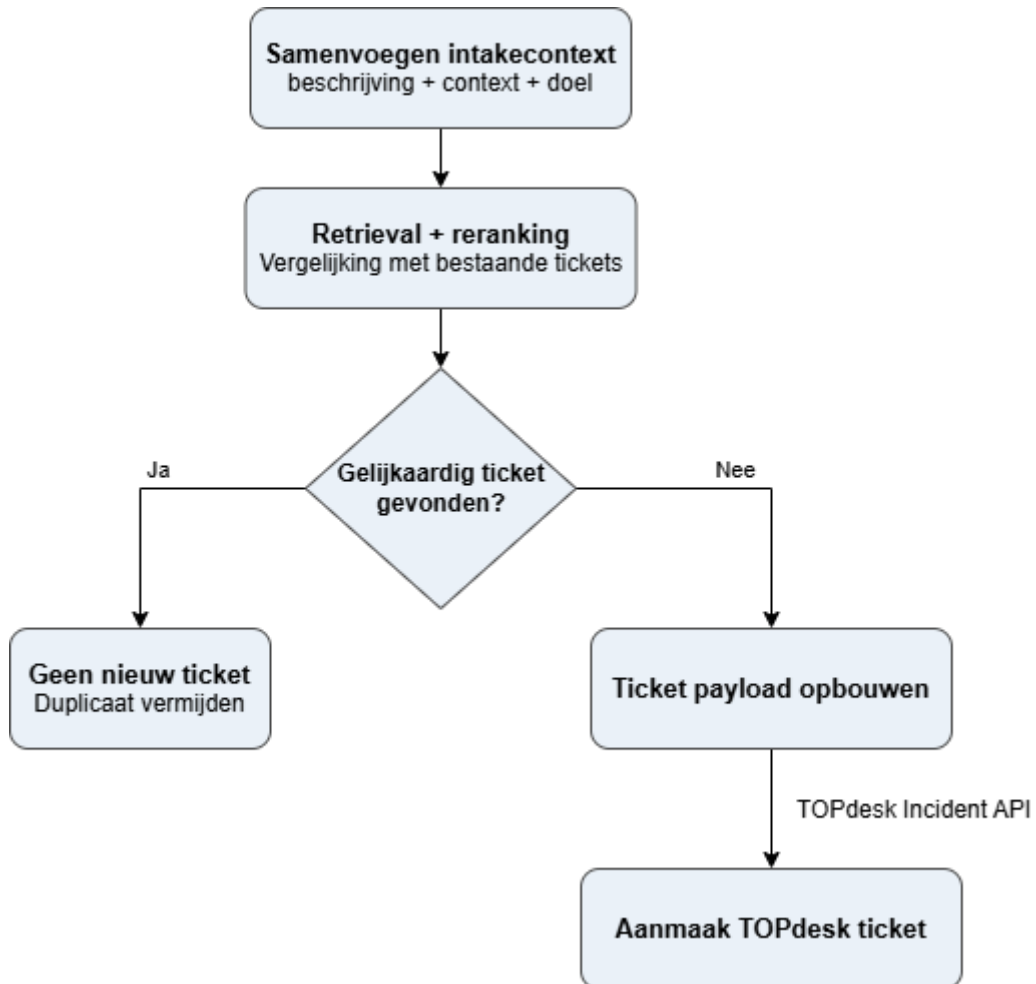
Figuur 26: Flow aanmaak ticket
