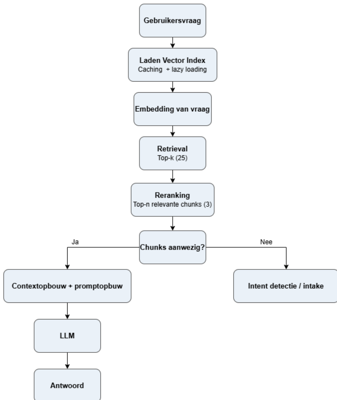
Figuur 15: Rag-pipeline
