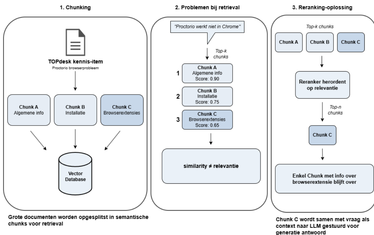
Figuur 3: Reranker als oplossing voor slechte retrieval
