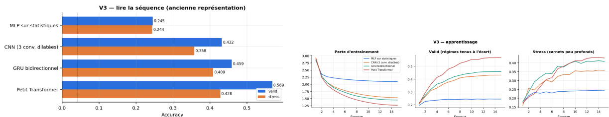
FIGURE 31 – Partie 3. Quatre réseaux sur l’ ancienne représentation relative. Lire la séquence plutôt que des résumés fait passer la valid de 0,245 (MLP sur statistiques) à 0,432 (CNN), 0,459 (GRU bidirectionnel) et 0,569 (petit Transformer). Même avec de mauvaises unités, l’ordre des événements porte beaucoup d’information.
