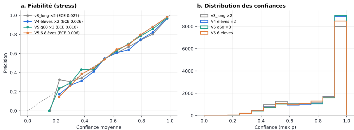
FIGURE 44 – Calibration sur le stress. (a) Courbes de fiabilité et erreur de calibration attendue (ECE, 12 classes de confiance). (b) Distribution des confiances.
