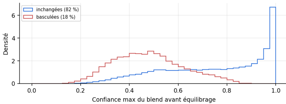
FIGURE 23 – 18 % des prédictions basculent. Leur confiance moyenne avant correction est de 0,48, contre 0,75 pour les fenêtres inchangées.
