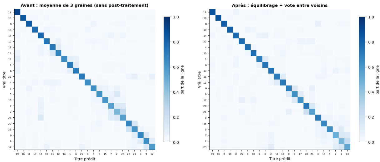
FIGURE 35 – Confusions du CNN simple sur le stress, avant (moyenne de 3 graines) et après (équilibrage + vote entre voisins). Les erreurs restantes se concentrent dans les mêmes familles que pour le grand modèle, \{20, 21\} , \{2, 7, 23\} , \{0, 9, 17\} : elles tiennent à la donnée plus qu’au modèle.
