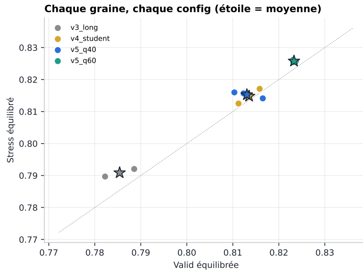
FIGURE 41 – Chaque graine, en valid et en stress équilibrés. Les générations forment des grappes nettes, et la dispersion entre graines (moins de 0,5 point) est petite devant l'écart entre générations.
