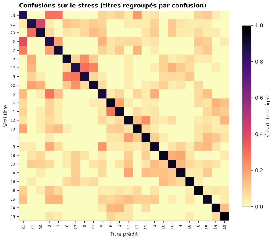
FIGURE 46 – Confusions de l’ensemble V5 sur le stress, avec les titres ordonnés par regroupement hiérarchique. Les erreurs ne sont pas diffuses : elles se concentrent dans quelques familles, notamment \{20, 21\} , \{2, 7, 23\} , \{0, 9, 17, 22\} et \{1, 6\} . À l’intérieur d’une famille, les titres partagent vraisemblablement un régime de tick et des conventions de lot proches (section 6). La séparation demande alors des traits plus fins que la grille de prix.
