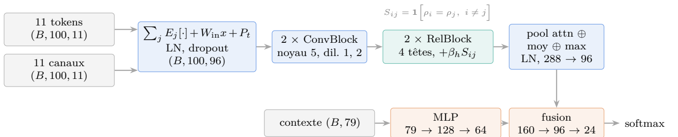
FIGURE 20 – Architecture de SignatureNet. En vert : le seul composant relationnel (le biais « même ordre »).
