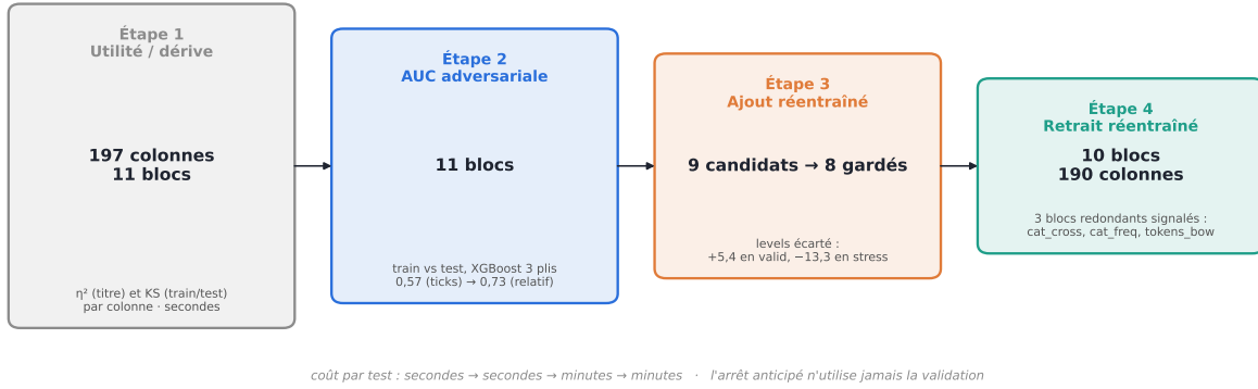
FIGURE 16 – L'entonnoir en quatre étapes, du moins cher au plus cher. Les deux premières étapes ne réentraînent rien : elles mesurent et localisent. Seules les deux dernières décident, en comparant des modèles réentraînés sur les mêmes fenêtres.
