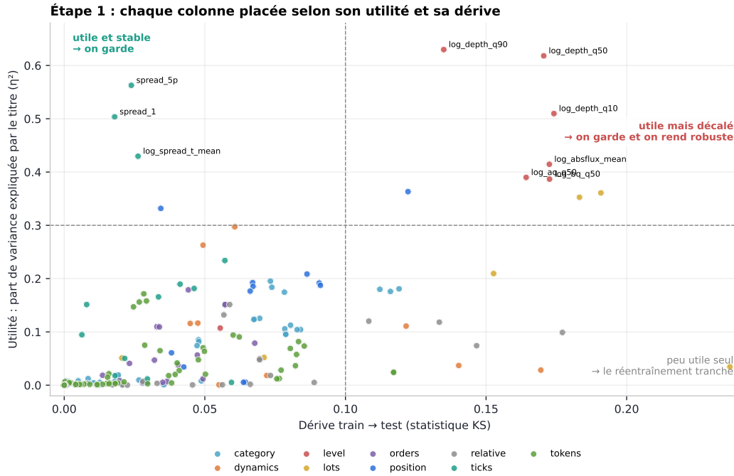
FIGURE 17 – Étape 1 sur les 197 colonnes du run 1. Les colonnes de tick (vert) occupent seules le quadrant idéal : \eta^2 \approx 0,5 pour une dérive KS \approx 0,02 . Les colonnes de profondeur (rouge) sont encore plus séparatrices, mais aussi les plus décalées : c'est le piège que l'étape 3 confirme. La majorité des colonnes sont peu utiles seules, ce qui ne dit rien de leur apport combiné.
