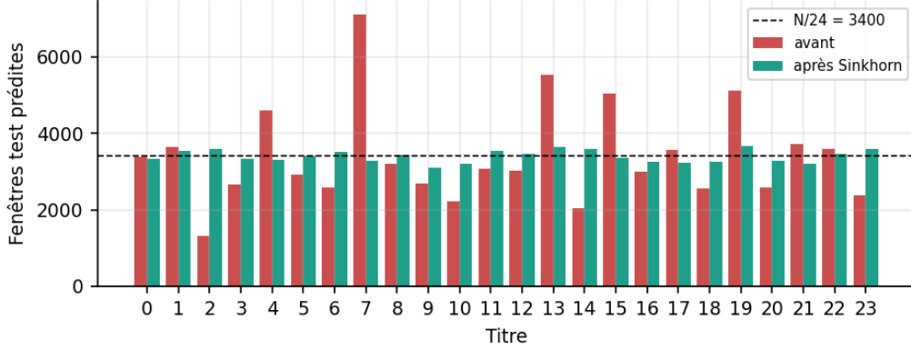
FIGURE 21 – Fenêtres test prédites par titre, avant et après équilibrage (blend des 4 finalistes, refit).
