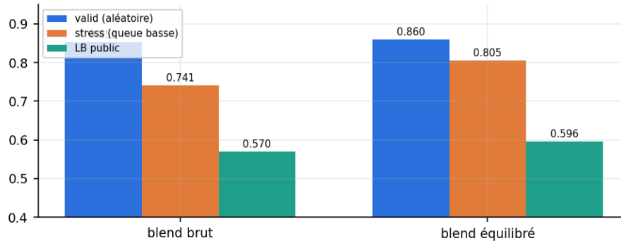
FIGURE 26 – Les trois mesures pour les deux soumissions. Le classement relatif (brut < équilibré) est le même partout. L'écart absolu, lui, ne l'est pas.
