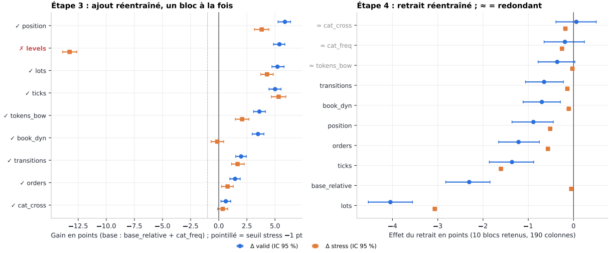
FIGURE 19 – Étapes 3 et 4 au run 1 (XGBoost, 50 % du fit, intervalles bootstrap appariés à 95 %). À gauche, l’ajout : huit blocs améliorent la validation et le stress. levels est le seul à violer la règle : +5,4 points en validation, -13,3 en stress. À droite, le retrait sur les 10 blocs retenus : lots , base_relative et ticks coûtent le plus cher. cat_cross , cat_freq et tokens_bow (≈) ont un intervalle qui contient 0 : ils sont redondants une fois les autres présents.
