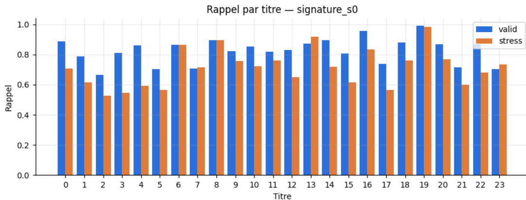
FIGURE 25 – Rappel par titre, signature_s0 .
