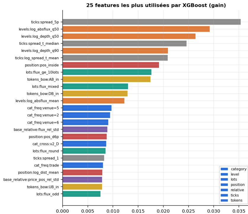
FIGURE 30 – Les 25 features les plus utilisées par XGBoost (gain). En tête, le spread en ticks ( ticks:spread_5p ), la signature stable, mais juste derrière, trois mesures de profondeur. Un arbre exploite tout ce qui sépare sur la période d’entraînement, sans distinguer signature et régime : c’est exactement ce que la figure 29 fait payer en stress.
