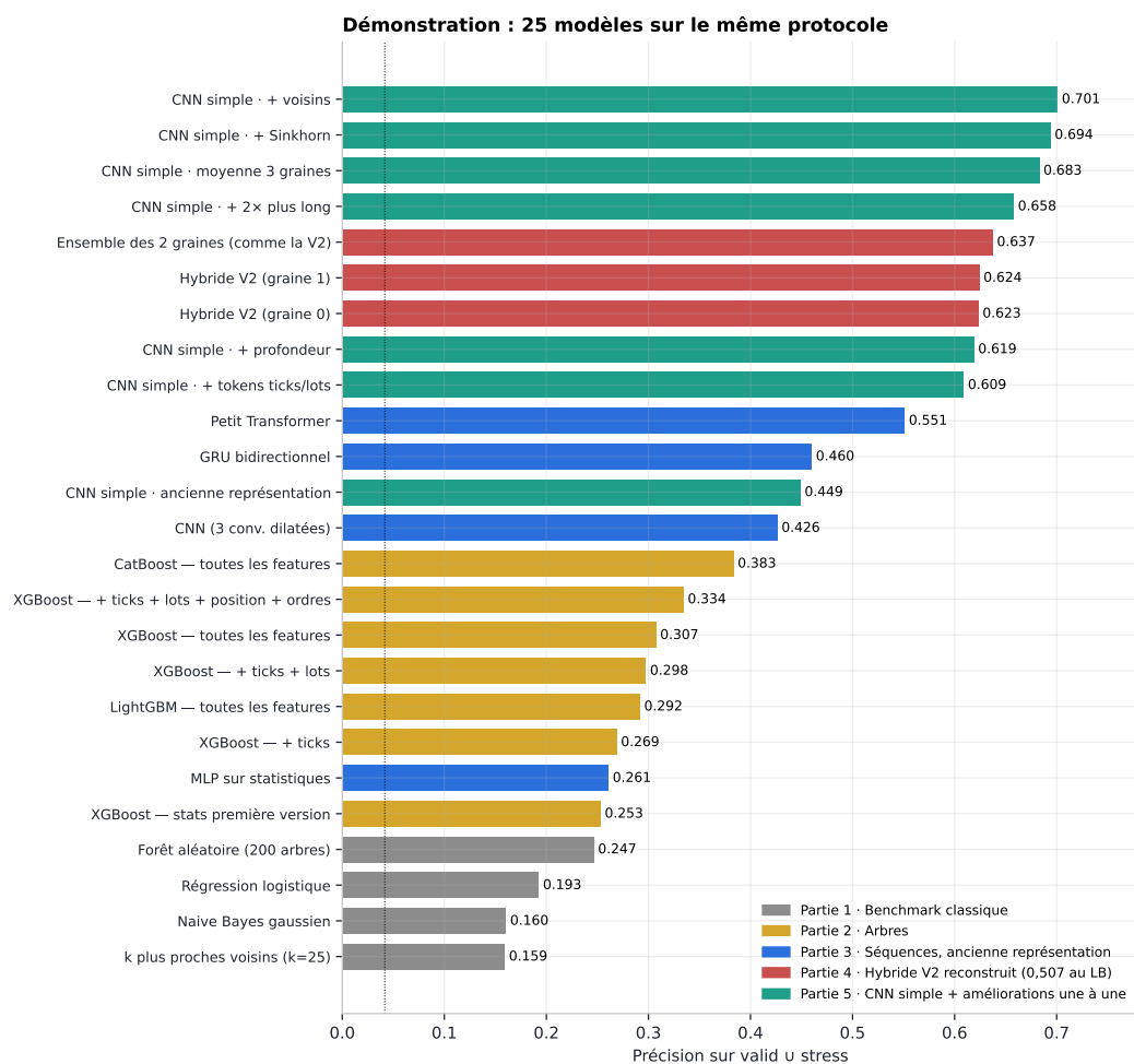
FIGURE 27 – Les 25 modèles du notebook, classés par précision sur valid \cup stress. Pour les parties 1 à 4, c'est la moyenne pondérée des précisions équilibrées valid et stress. Pour la partie 5, c'est la précision mesurée directement sur l'union (équilibrée à partir de l'étape Sinkhorn). Un petit CNN d'environ 100 k paramètres, nourri des tokens en ticks et en lots, dépasse la reconstruction de l'ancien meilleur modèle dès qu'on l'entraîne plus longtemps.
