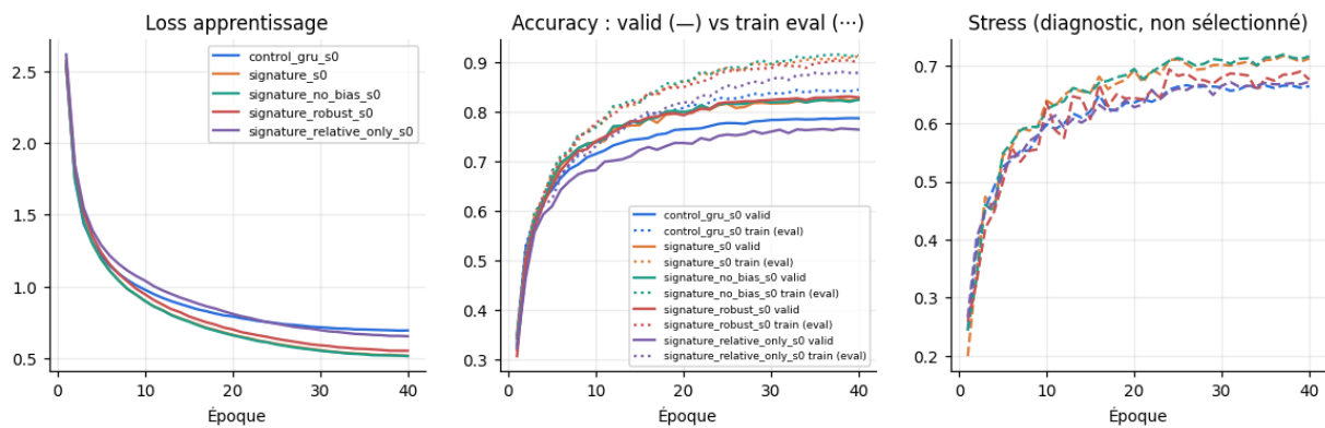
FIGURE 24 – Courbes d’apprentissage (seed 0). Le stress est tracé mais ne sélectionne rien.
