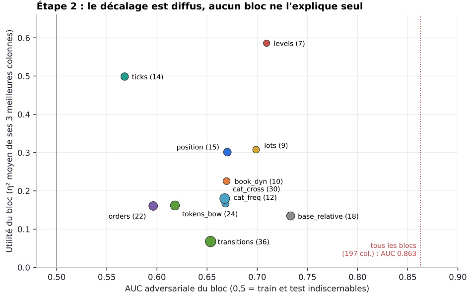
FIGURE 18 – Étape 2 : chaque bloc placé selon son décalage (AUC adversariale) et son utilité (taille du point = nombre de colonnes). Les blocs s'étalent de 0,57 ( ticks ) à 0,73 ( base_relative , les résumés de l'ancien pipeline), mais tous ensemble atteignent 0,863 : le décalage est diffus, réparti entre de nombreuses colonnes. Fait notable, les résumés relatifs, pensés pour être invariants à l'échelle, sont les plus décalés.
