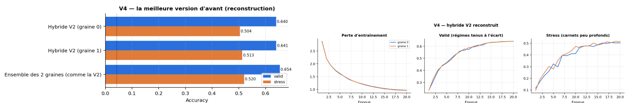
FIGURE 32 – Partie 4. Reconstruction simplifiée du Transformer hybride de la V2, le record historique à 0,507 au LB. Deux graines donnent 0,640–0,641 en valid et 0,504–0,513 en stress, l’ensemble 0,654 et 0,520. Fait notable : le stress brut de ce modèle (0,52) est très proche de son score public (0,507), alors que la valid le surestime de 15 points.
