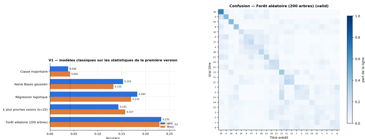
FIGURE 28 – Partie 1. Modèles classiques sur les statistiques de fenêtre de la toute première version. Le meilleur, une forêt aléatoire, plafonne à 0,23 en valid et 0,25 en stress, avec une confusion diffuse : ces statistiques ne portent presque pas la signature des titres.
