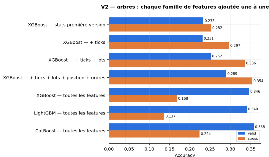
FIGURE 29 – Partie 2. XGBoost en ajoutant une famille de features à la fois. Les familles stables font monter le stress à chaque ajout : 0,252 (statistiques initiales), 0,297 (+ ticks), 0,336 (+ lots), 0,354 (+ position et ordres). Avec toutes les features, profondeur comprise, la valid monte à 0,346 mais le stress s'effondre à 0,168 (0,137 pour LightGBM, 0,224 pour CatBoost). C'est le piège de régime de la section 11, reproduit ici sur trois implémentations différentes.
