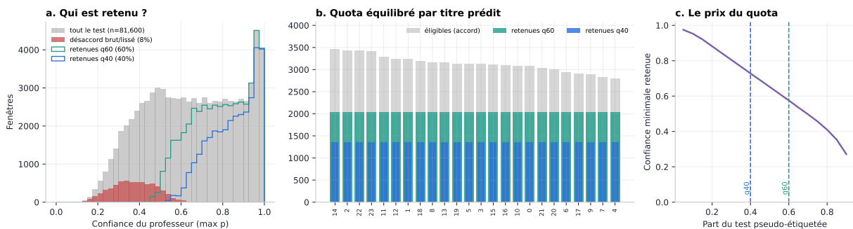
FIGURE 39 – Sélection des pseudo-labels V5. (a) Les fenêtres où les deux lectures divergent ont une confiance faible (mode vers 0,3) : le filtre écarte bien les cas douteux. (b) Le quota coupe les titres sur-prédits : chaque titre reçoit exactement 2 040 (resp. 1 360) fenêtres. (c) Confiance minimale atteinte si l'on étendait la sélection sans quota. Elle chute rapidement au-delà de 60 %, ce qui borne l'intérêt d'aller plus loin.
