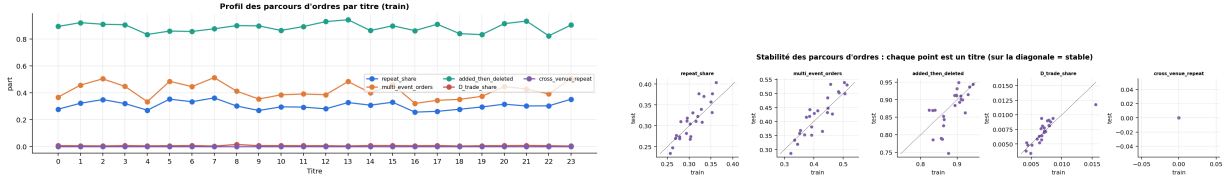
FIGURE 13 – À gauche, des profils de parcours d'ordres par titre : part d'ordres ajoutés puis supprimés dans la fenêtre (83 à 94 %), part d'ordres à plusieurs événements (33 à 50 %), part de répétitions. Les ordres exécutés sont rares. À droite, chaque point est un titre, train en abscisse et test en ordonnée. Les points restent proches de la diagonale : contrairement à la profondeur, la façon dont les ordres vivent et meurent est stable d'une période à l'autre.
