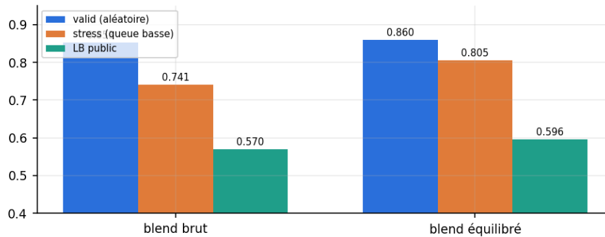
FIGURE 24 – Les trois mesures pour les deux soumissions. Le classement relatif (brut < équilibré) est le même partout. L'écart absolu, lui, ne l'est pas.
