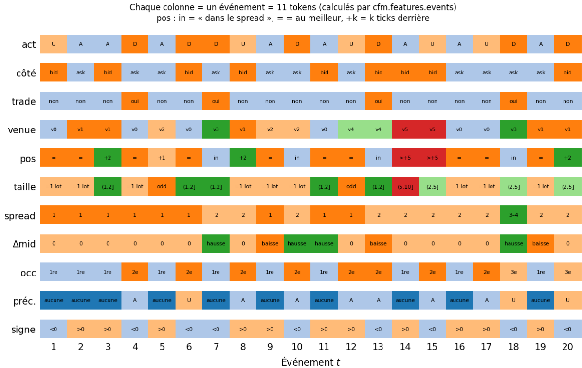
FIGURE 15 – La même information en bandeau : une colonne par événement, une ligne par token. C’est littéralement ce que voit SignatureNet avant ses couches d’embedding.
