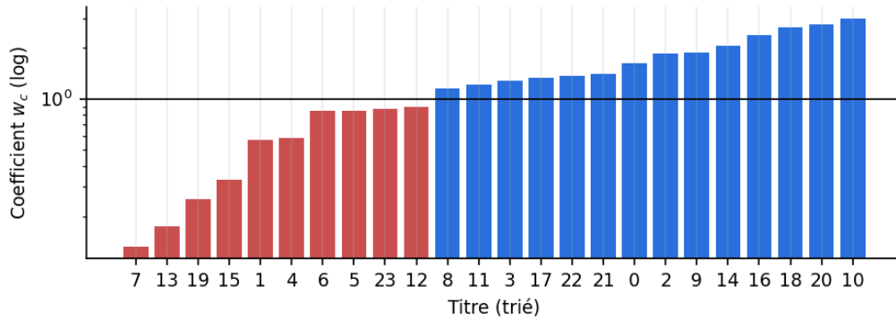
FIGURE 18 – Coefficients w_k (normalisés en moyenne géométrique). Titre 7 : \times 0,13 ; titre 10 : \times 2,99 .
