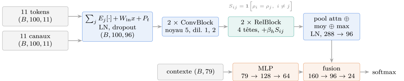
FIGURE 16 – Architecture de SignatureNet. En vert : le seul composant relationnel (le biais « même ordre »).
