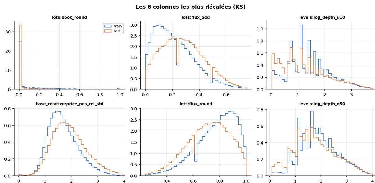
FIGURE 11 – Les six colonnes les plus décalées entre train (bleu) et test (orange), au sens du test de Kolmogorov–Smirnov. Toutes appartiennent aux familles lots et profondeur : moins de lots ronds, plus d’odd lots, des carnets moins profonds. Aucune colonne de tick n’y figure.
