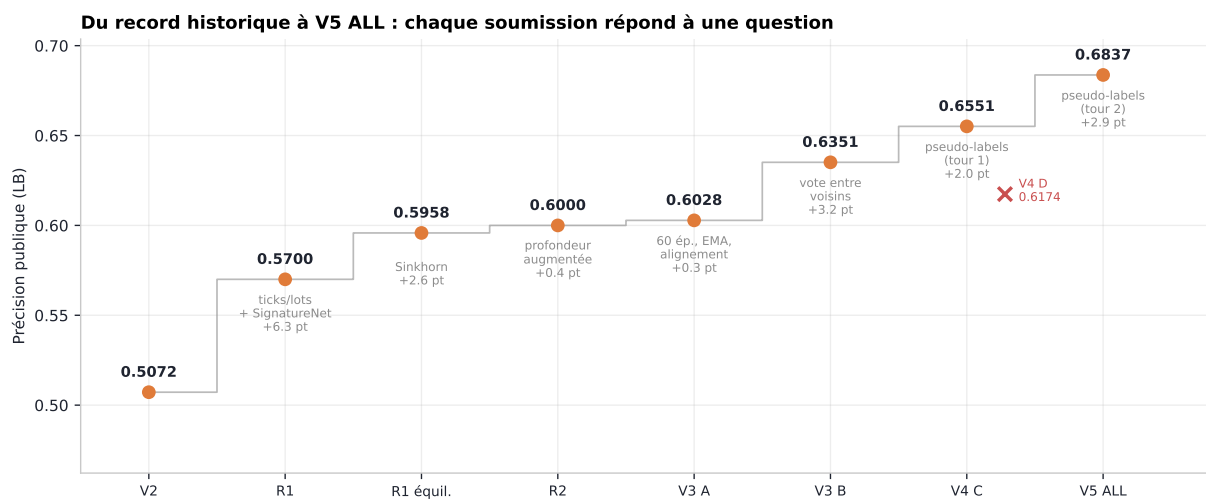
FIGURE 1 – Accuracy publique, soumission par soumission, avec le levier ajouté à chaque étape. La croix rouge est une soumission de contrôle (V4 D : V4 C sans les élèves). Section 18 pour V4 et V5.
