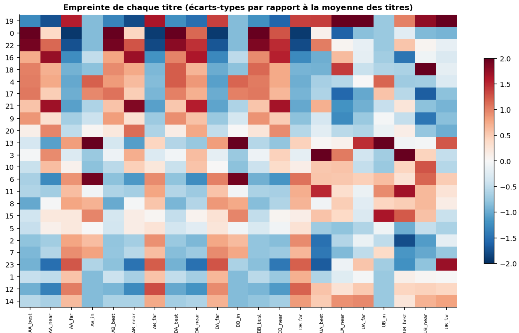
FIGURE 10 – L’empreinte « sac de mots » de chaque titre : fréquence des combinaisons action \times côté \times zone de prix, en écarts-types par rapport à la moyenne des titres. Les titres sont réordonnés par ressemblance. Des blocs de titres aux empreintes voisines apparaissent, par exemple 0 et 22, et ces familles se retrouvent dans les matrices de confusion (figure 44, famille \{0, 9, 17, 22\} ).
