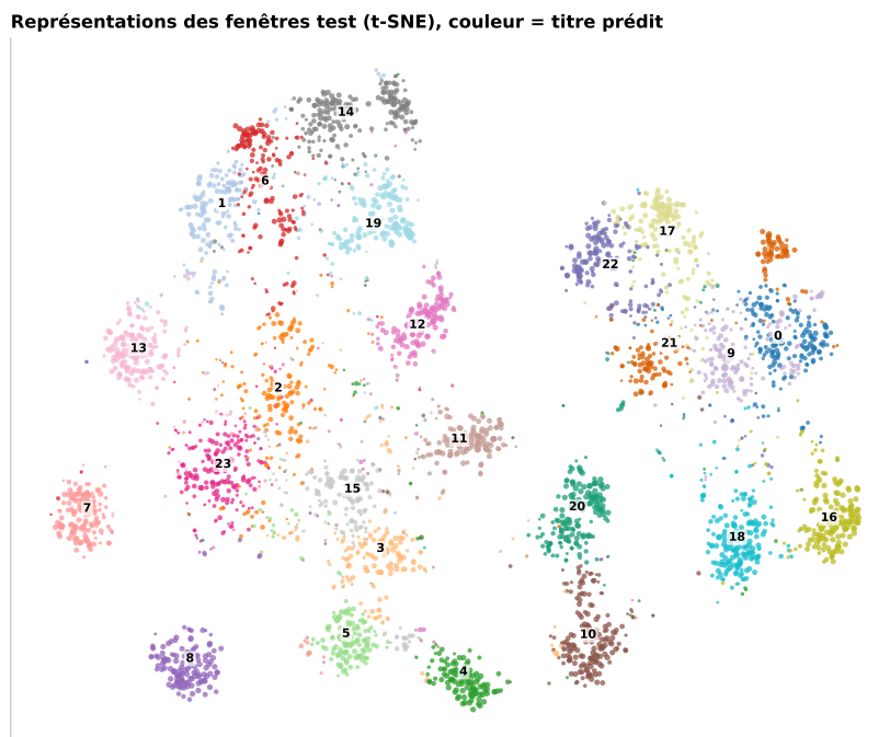
FIGURE 45 – Carte t-SNE de 4000 fenêtres test (représentations des élèves V5 refit), couleur = titre prédit, taille = confiance. Plusieurs titres forment des îlots isolés (7, 8, 13, 16). D'autres se touchent, et ce sont les mêmes familles que sur la matrice de confusion : \{0, 9, 17, 21, 22\} à droite, \{1, 6, 14, 19\} en haut.
