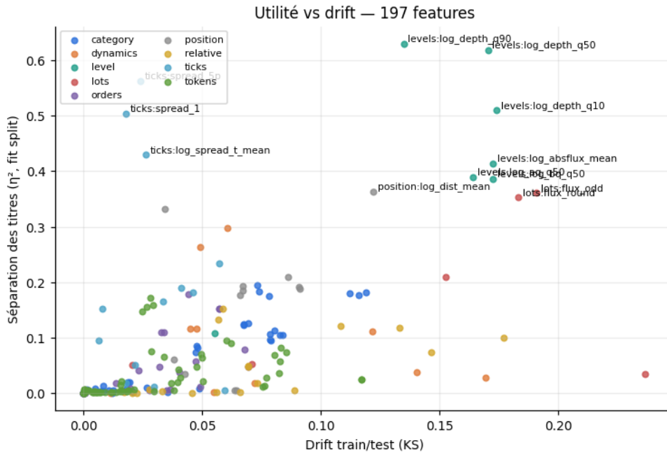
FIGURE 20 – Carte utilité/dérive des 197 colonnes.
