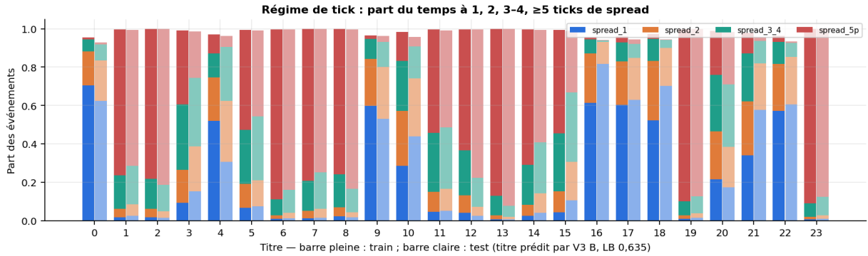
FIGURE 6 – Part du temps passé avec un spread de 1, 2, 3-4 ou au moins 5 ticks, par titre (barre pleine : train ; barre claire : test). Les titres se rangent en deux familles nettes : ceux qui vivent à un tick (0, 9, 16, 17, 22...) et ceux dont le spread dépasse presque toujours 5 ticks. Les barres train et test sont presque identiques : c'est la signature stable par excellence ( KS \approx 0,02 , section 16).
