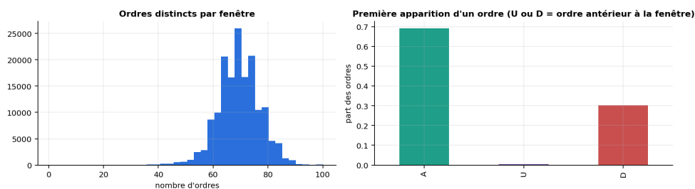
FIGURE 5 – Ordres par fenêtre. À gauche, une fenêtre de 100 événements touche environ 70 ordres distincts : la plupart n’apparaissent qu’une fois, mais un tiers environ reviennent. À droite, la première apparition d’un ordre est un ajout dans 70 % des cas, et une suppression dans 30 % : ces ordres ont été placés avant la fenêtre. D’où l’intérêt des tokens d’occurrence et d’action précédente du même ordre (section 7).
