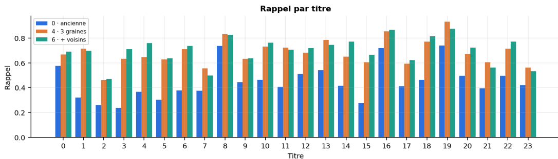
FIGURE 34 – Rappel par titre : ancienne représentation (étape 0), 3 graines (étape 4), après voisins (étape 6). Le gain est général, il ne vient pas de quelques titres faciles. Les plus gros sauts concernent des titres que l'ancienne représentation ne reconnaissait presque pas (1, 3, 5, 15 : de 0,25–0,3 à plus de 0,6).
