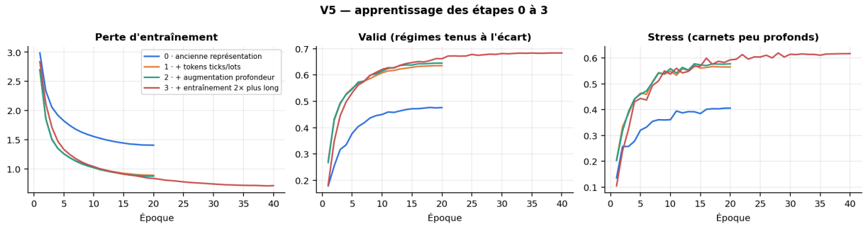
FIGURE 32 – Courbes d'apprentissage des étapes 0 à 3. L'ancienne représentation (bleu) plafonne vers 0,47 en valid. Toutes les variantes à tokens montent plus vite et plus haut. L'entraînement long (rouge) continue de progresser jusqu'à l'époque 40.
