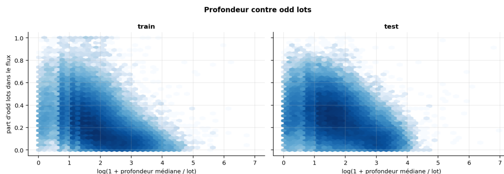
FIGURE 12 – Part d’odd lots en fonction de la profondeur, train contre test. La relation est décroissante dans les deux périodes, et le nuage du test glisse vers les carnets moins profonds et plus riches en odd lots. Un même mécanisme, des prix plus élevés, expliquerait les deux décalages à la fois : à valeur égale, moins d’actions par ordre.
