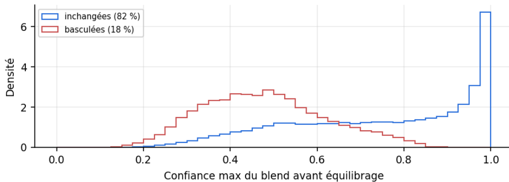
FIGURE 19 – 18 % des prédictions basculent. Leur confiance moyenne avant correction est de 0,48, contre 0,75 pour les fenêtres inchangées.
