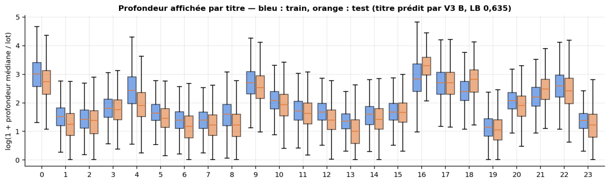
FIGURE 8 – Profondeur médiane du carnet (log, en lots) par titre, train en bleu et test en orange. Elle sépare bien les titres, mais elle baisse sur le test pour la majorité d'entre eux. C'est le piège de régime de la section 11, et la motivation de l'augmentation et de l'alignement de profondeur.
