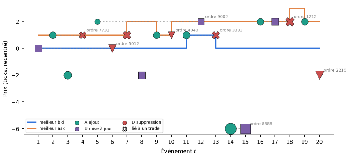
FIGURE 14 – Le motif en image. Les escaliers sont les meilleures limites ; chaque marqueur est un événement (couleur = action, croix = lié à un trade, taille \propto \sqrt{|f|} ). Les pointillés relient les événements d'un même ordre : ce sont les parcours que les tokens d'occurrence et d'action précédente encodent.
