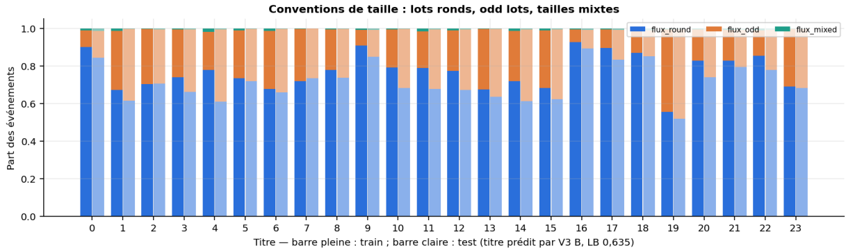
FIGURE 7 – Répartition du flux entre lots ronds (multiples de 100), odd lots et tailles mixtes. Les titres se distinguent nettement par leurs conventions de taille. Mais sur la période test, la part d'odd lots augmente pour presque tous les titres. C'est un premier indice de prix plus élevés (section 13.4).
