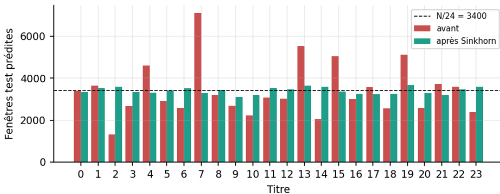
FIGURE 17 – Fenêtres test prédites par titre, avant et après équilibrage (blend des 4 finalistes, refit).
