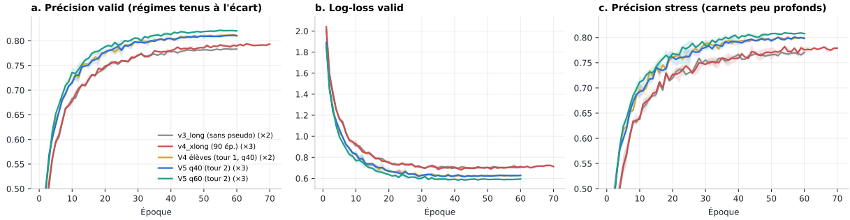
FIGURE 38 – Courbes d'apprentissage des trois générations (moyenne sur les graines ; bande = min/max). Les élèves des deux tours se séparent des modèles sans pseudo-labels dès les premières époques. Leur log-loss valid descend à 0,59–0,63 contre 0,70 et ne remonte pas. v4_xlong rejoint v3_long sans le dépasser nettement (la courbe s'arrête à 70 époques, l'arrêt précoce d'une graine).
