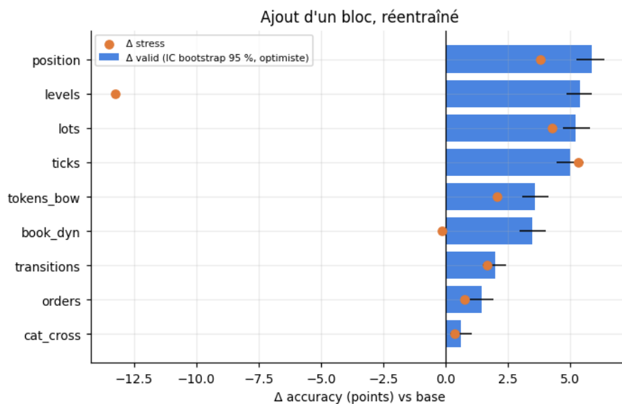
FIGURE 21 – Ajout réentraîné, valid et stress.
