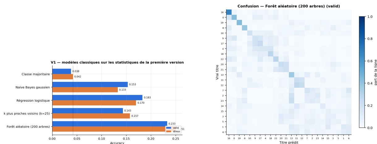
FIGURE 26 – Partie 1. Modèles classiques sur les statistiques de fenêtre de la toute première version. Le meilleur, une forêt aléatoire, plafonne à 0,23 en valid et 0,25 en stress, avec une confusion diffuse : ces statistiques ne portent presque pas la signature des titres.
