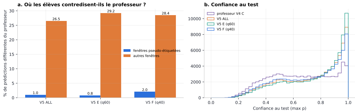
FIGURE 41 – (a) Désaccords avec le professeur, sur et hors pseudo-labels. (b) Confiance au test. La masse du professeur, étalée entre 0,4 et 0,7, se concentre chez les élèves au-dessus de 0,9.
