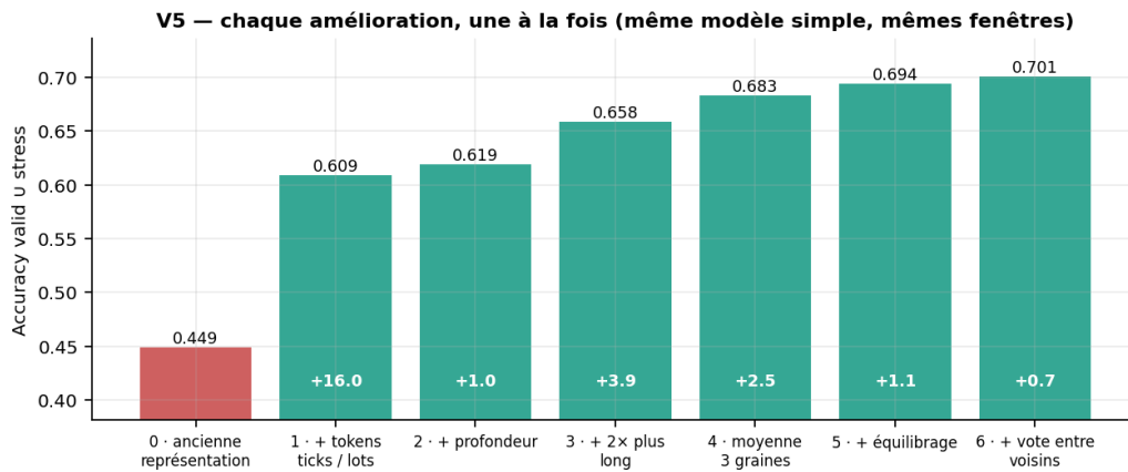
FIGURE 31 – L'échelle de la table 20 en image. À comparer avec la progression publique de la figure 1 : les leviers arrivent dans le même ordre d'importance, à une exception près. Le vote entre voisins rapporte peu en interne (+0,7) et beaucoup au LB (+3,2), parce que le test contient quatre fois plus de fenêtres par titre-jour que le pool.
