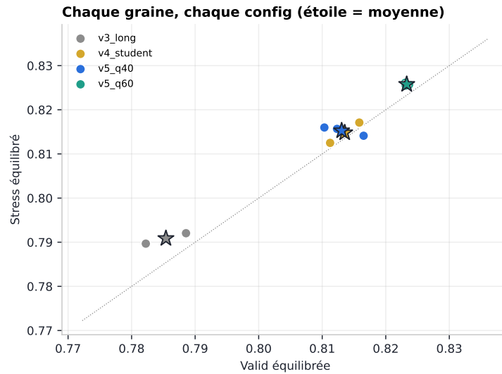
FIGURE 39 – Chaque graine, en valid et en stress équilibrés. Les générations forment des grappes nettes, et la dispersion entre graines (moins de 0,5 point) est petite devant l'écart entre générations.
