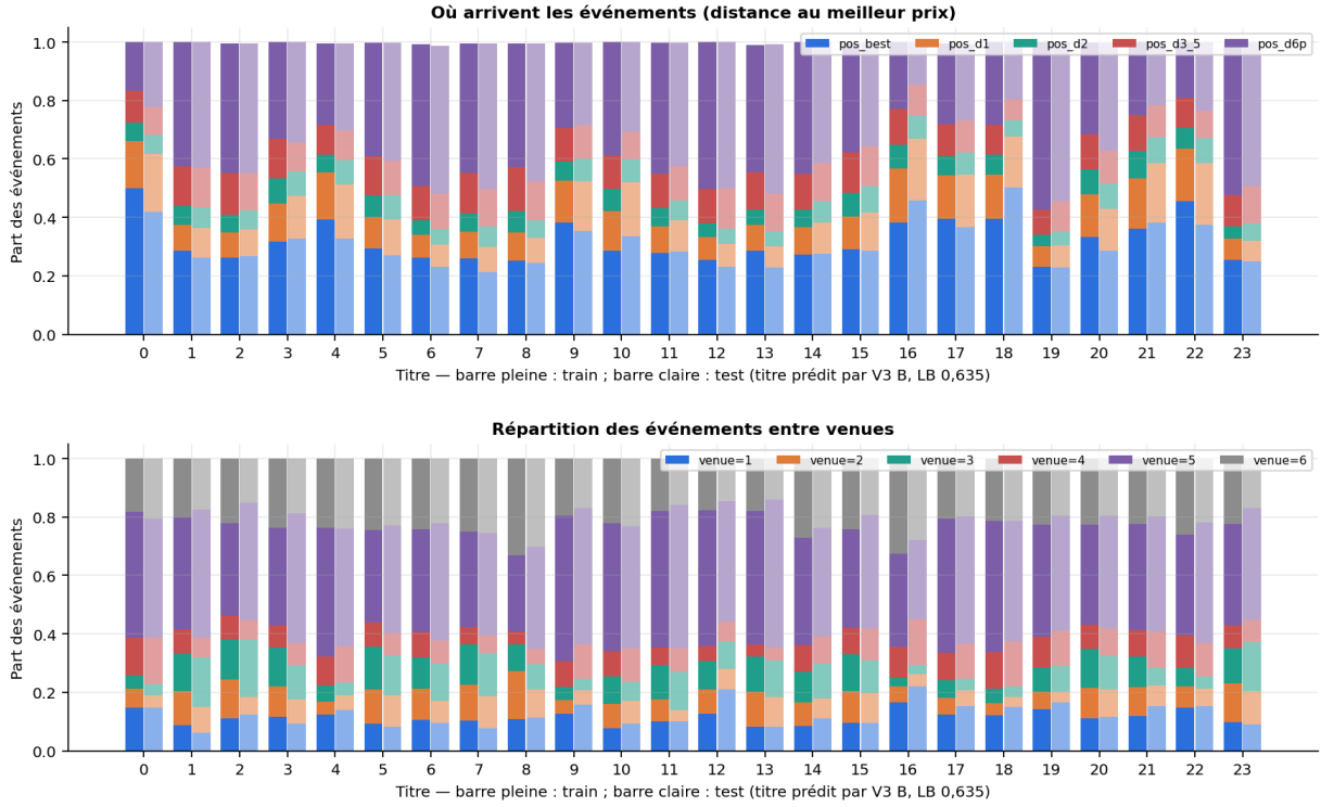
FIGURE 9 – En haut, la distance des événements au meilleur prix (au meilleur, à 1, 2, 3-5, 6 ticks et plus). En bas, la répartition entre venues. Les deux varient d'un titre à l'autre et restent stables entre train et test : ce sont des signatures secondaires, mais fiables.
