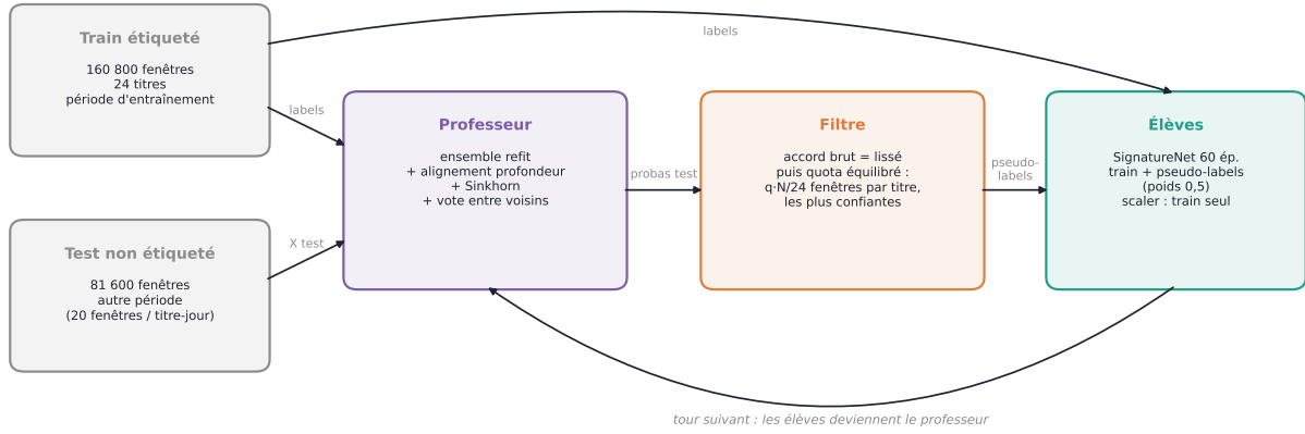
FIGURE 36 – La boucle d’auto-apprentissage. Le professeur étiquette les fenêtres test où ses deux lectures concordent ; un quota par titre empêche de transmettre son biais de classes ; les élèves s’entraînent sur \text{train} \cup \text{pseudo-labels} , puis deviennent le professeur du tour suivant.
