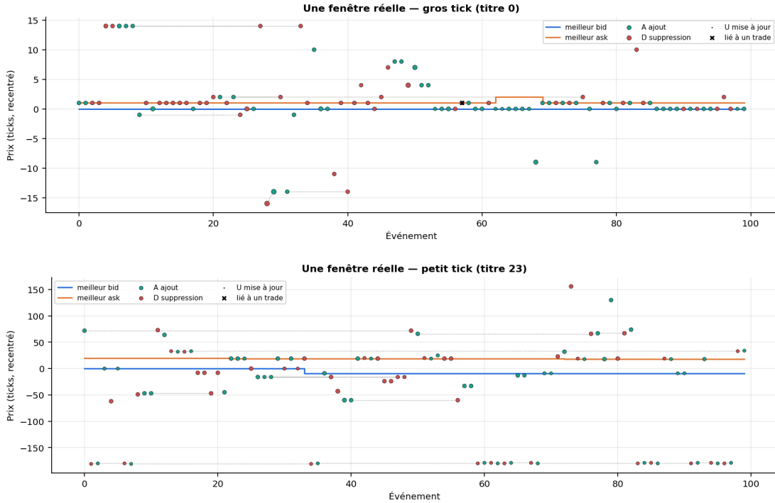
FIGURE 3 – Deux vraies fenêtres de 100 événements, prix en ticks recentrés sur le mid initial. En haut, un titre à gros tick (titre 0) : le meilleur bid et le meilleur ask sont collés à un tick d'écart et ne bougent presque pas, et les ordres se placent sur quelques niveaux entiers. En bas, un titre à petit tick (titre 23) : les ordres s'étalent sur \pm 150 ticks et le spread vaut plusieurs dizaines de ticks. Exprimées en multiples d'une médiane locale, ces deux fenêtres se ressembleraient bien davantage. C'est l'argument visuel de la section 6.
