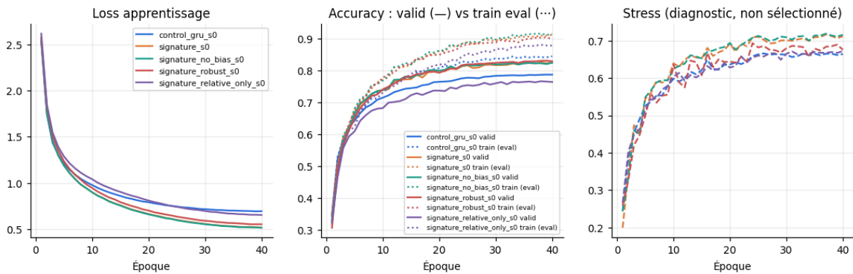
FIGURE 22 – Courbes d’apprentissage (seed 0). Le stress est tracé mais ne sélectionne rien.
