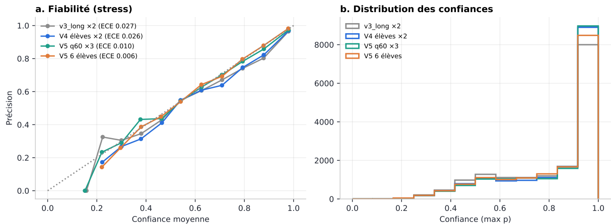
FIGURE 42 – Calibration sur le stress. (a) Courbes de fiabilité et erreur de calibration attendue (ECE, 12 classes de confiance). (b) Distribution des confiances.
