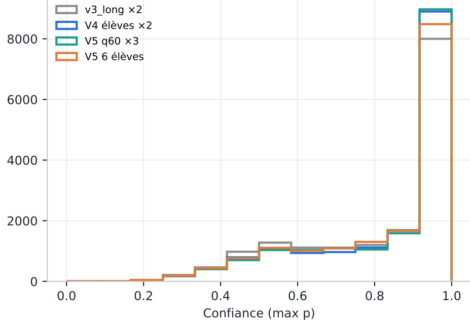
b. Distribution des confiances
