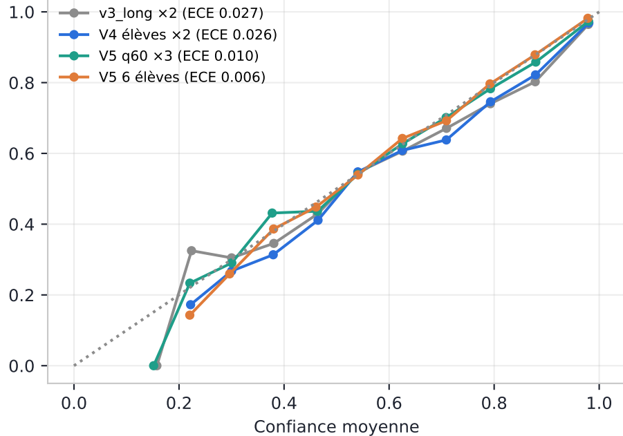
a. Fiabilité (stress)
