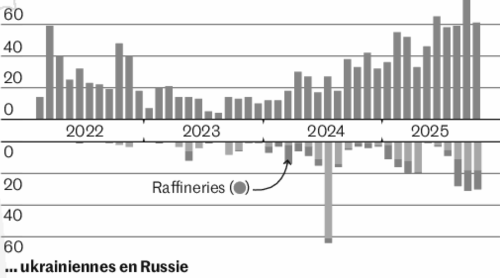
Frappes contre des infrastructures énergétiques, par mois...
