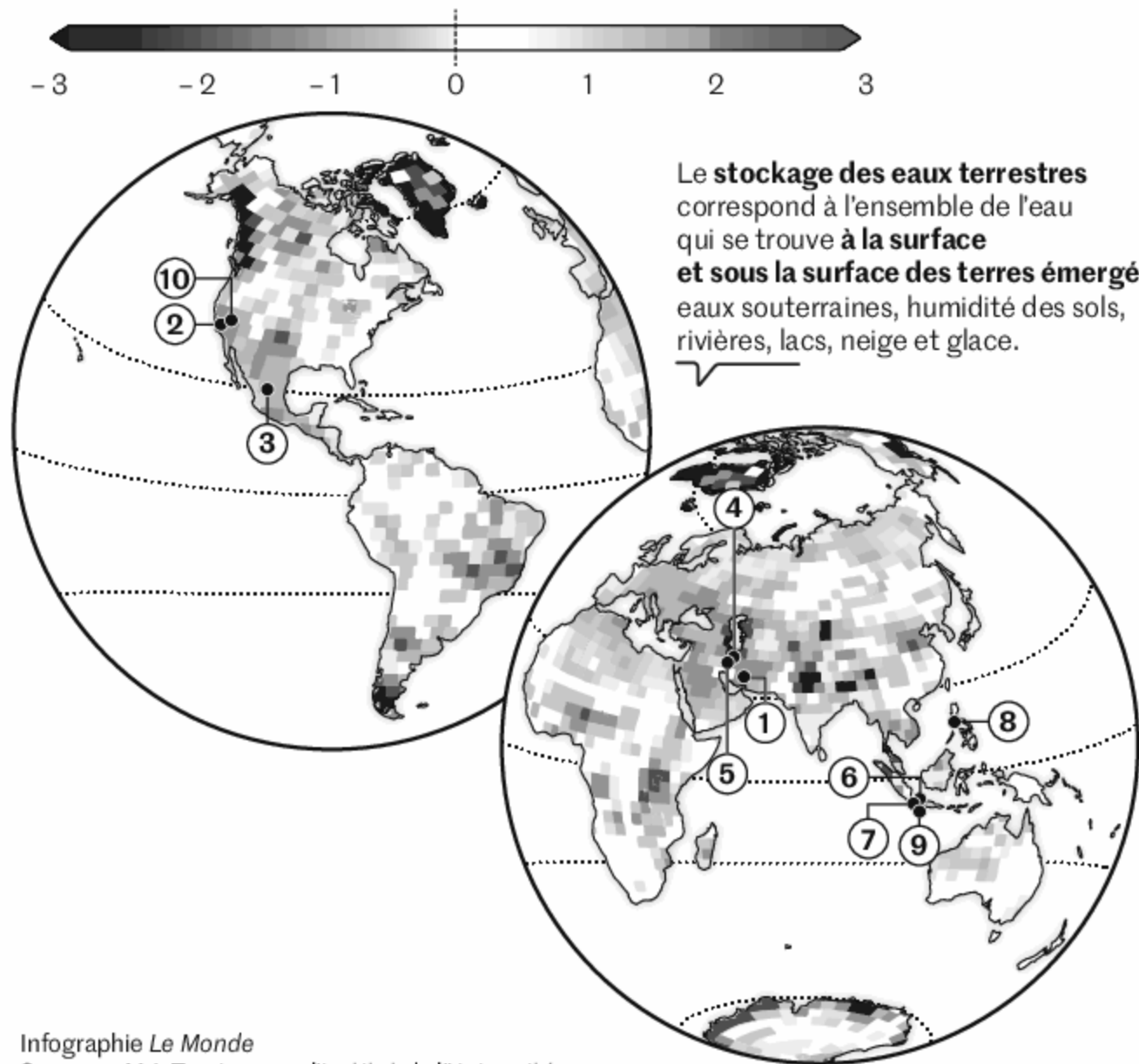
Evolution des capacités de stockage des eaux terrestres*, entre avril 2002 et septembre 2025, en centimètres par an
