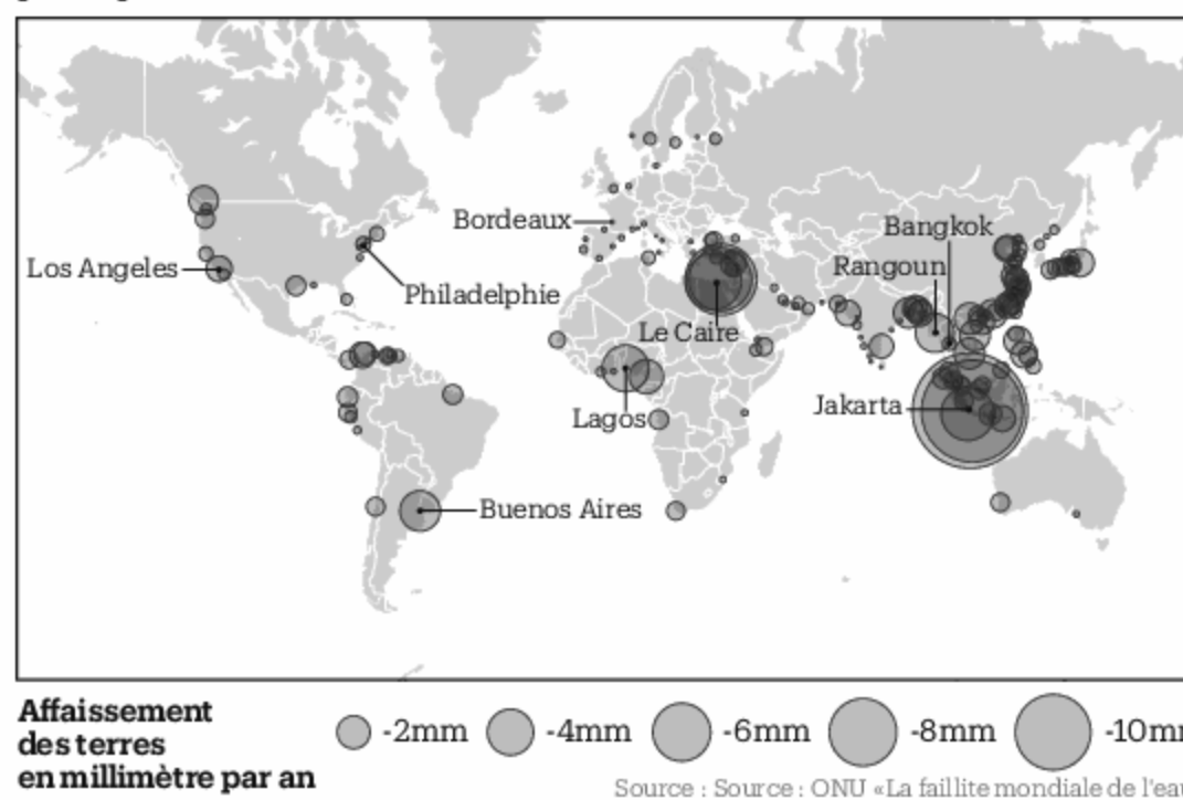
L'affaissement des sols sur les côtes Affaissement des sols dans 204 villes côtières du monde, principalement dû à l'extraction des eaux souterraines, de 2015 à 2024
