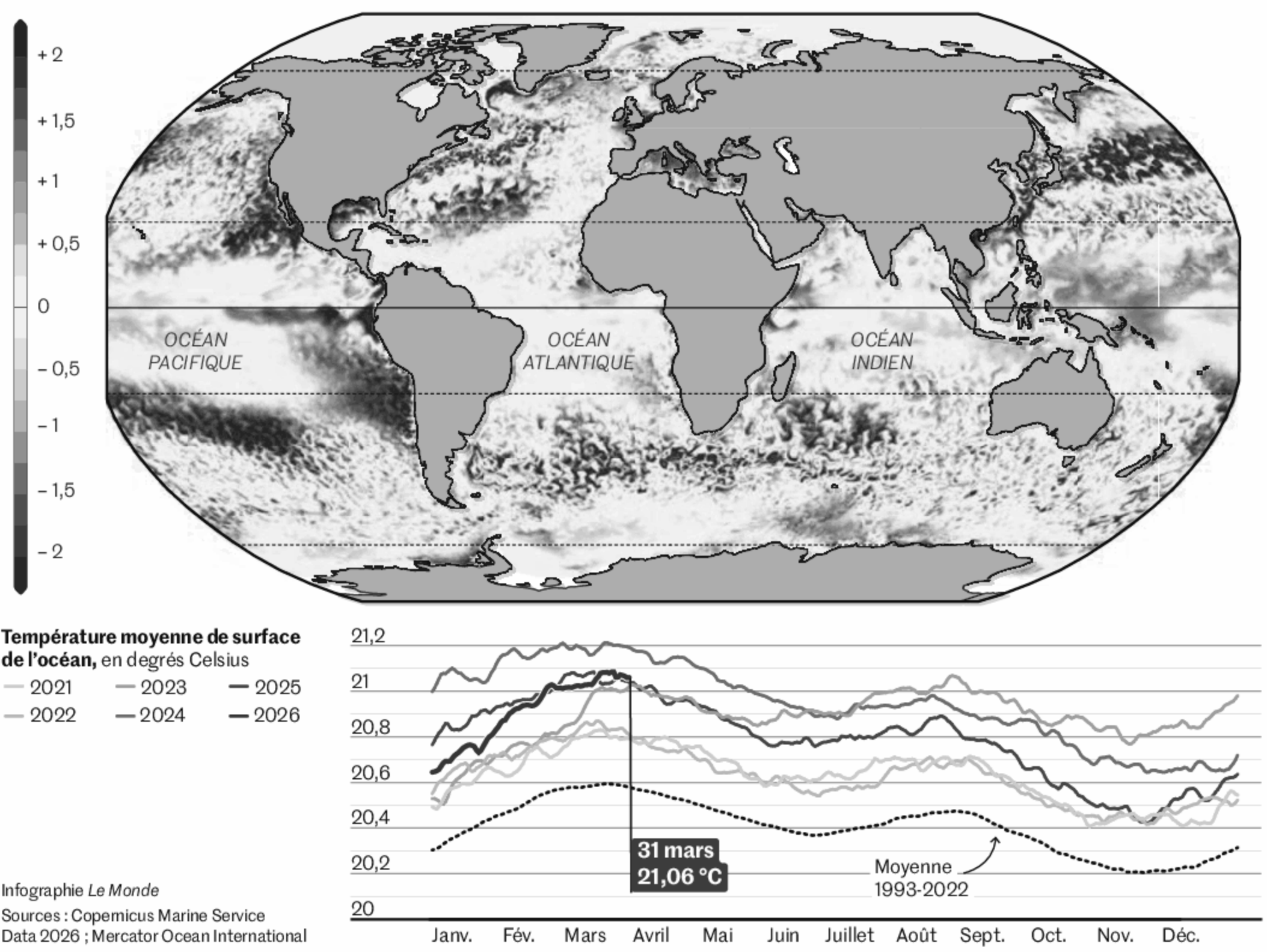
Anomalies de température de surface en mars 2026, en degrés Celsius, par rapport à la moyenne 1993-2022
