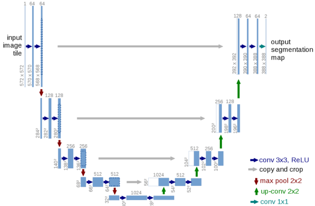
Hình 2.2: Kiến trúc U-Net với bốn cấp độ phân giải.
