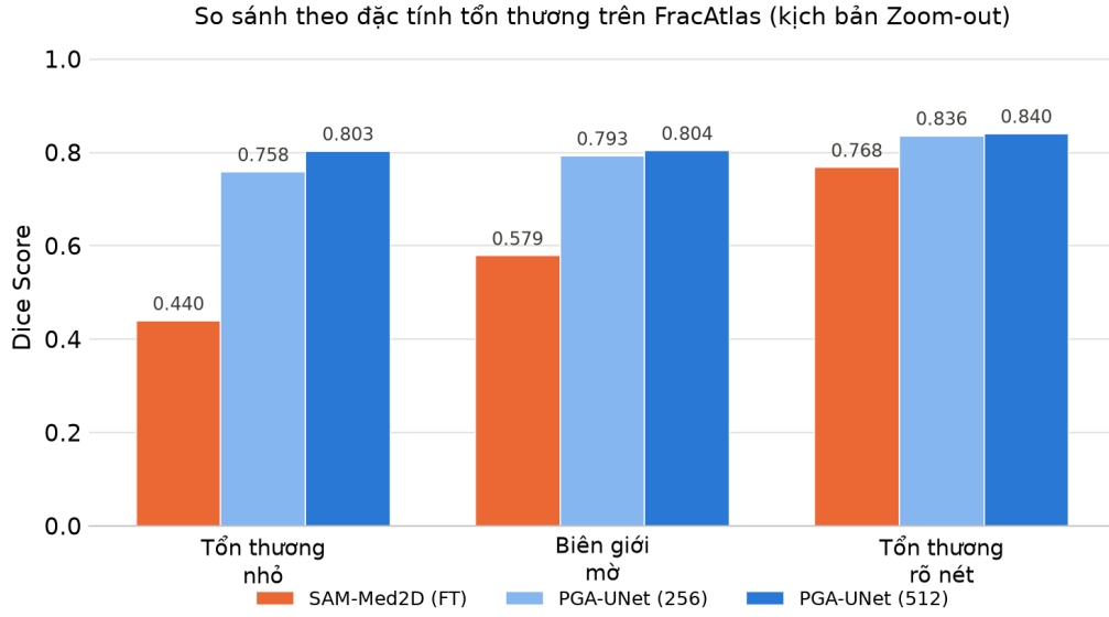
Hình 4.6: So sánh SAM-Med2D (FT), PGA-UNet (256) và PGA-UNet (512) theo ba nhóm đặc tính tổn thương trên FracAtlas (Bảng 4.19).
