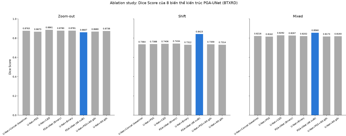
Hình 4.2: Ablation study: Dice Score của 8 biến thể kiến trúc PGA-UNet trên ba kịch bản câu nhắc (Bảng 4.7). PGA-UNet (đề xuất) tô xanh dương, các biến thể còn lại tô xám.
