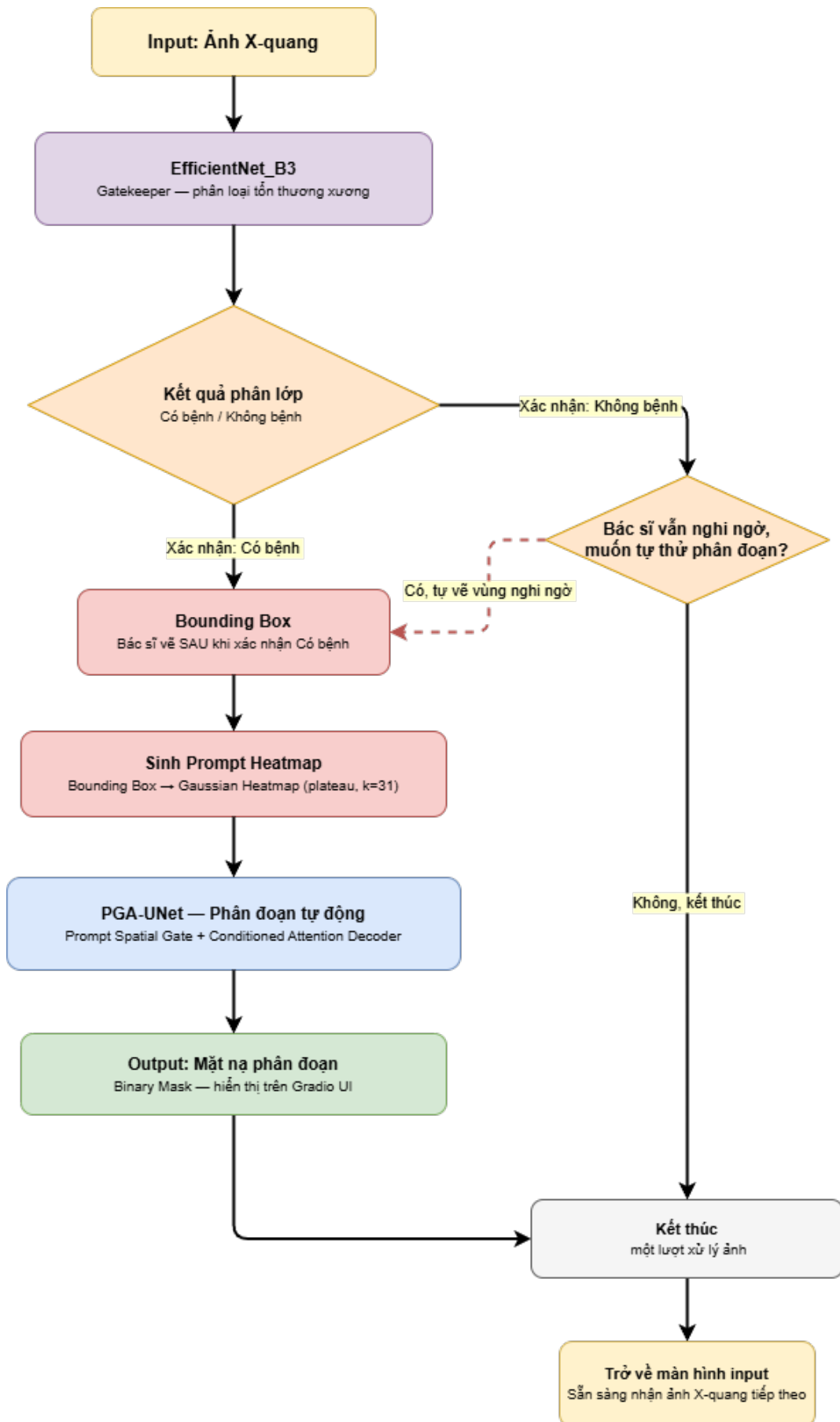
Hình 3.1: Luồng xử lý tổng thể hệ thống: ảnh X-quang qua EfficientNet_B3 để sinh gợi ý sàng lọc; bác sĩ xem gợi ý và xác nhận (không bệnh → kết thúc, có bệnh → vẽ hộp giới hạn) trước khi hệ thống chuyển sang PGA-UNet phân đoạn có hướng dẫn.
