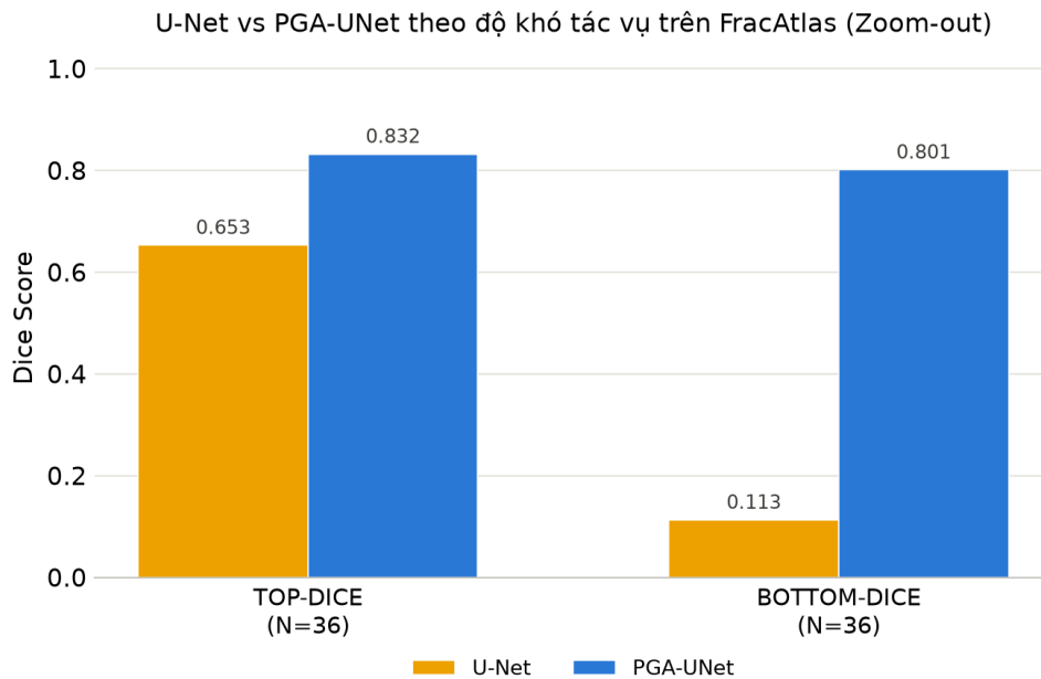
Hình 4.5: So sánh U-Net và PGA-UNet theo độ khó tác vụ trên FracAtlas (Bảng 4.18).
