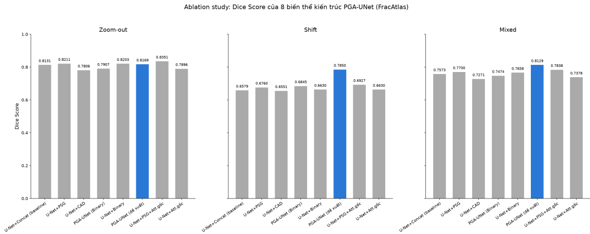
Hình 4.7: Ablation study: Dice Score của 8 biến thể kiến trúc PGA-UNet trên ba kịch bản câu nhắc trên FracAtlas (Bảng 4.20). PGA-UNet (đề xuất) tô xanh dương, các biến thể còn lại tô xám.
