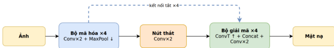
Hình 2.2: Kiến trúc U-Net với bốn cấp độ phân giải.
