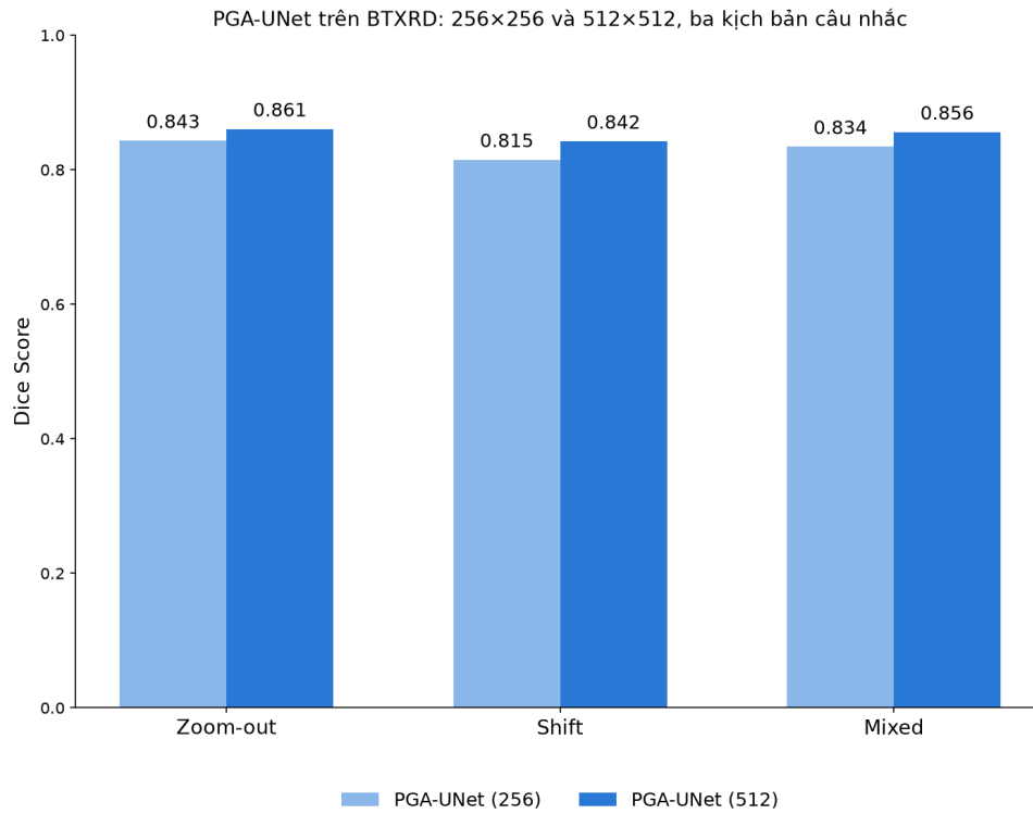
Hình 4.4: PGA-UNet trên BTXRD: 256×256 và 512×512, ba kịch bản câu nhắc (Bảng 4.8).
