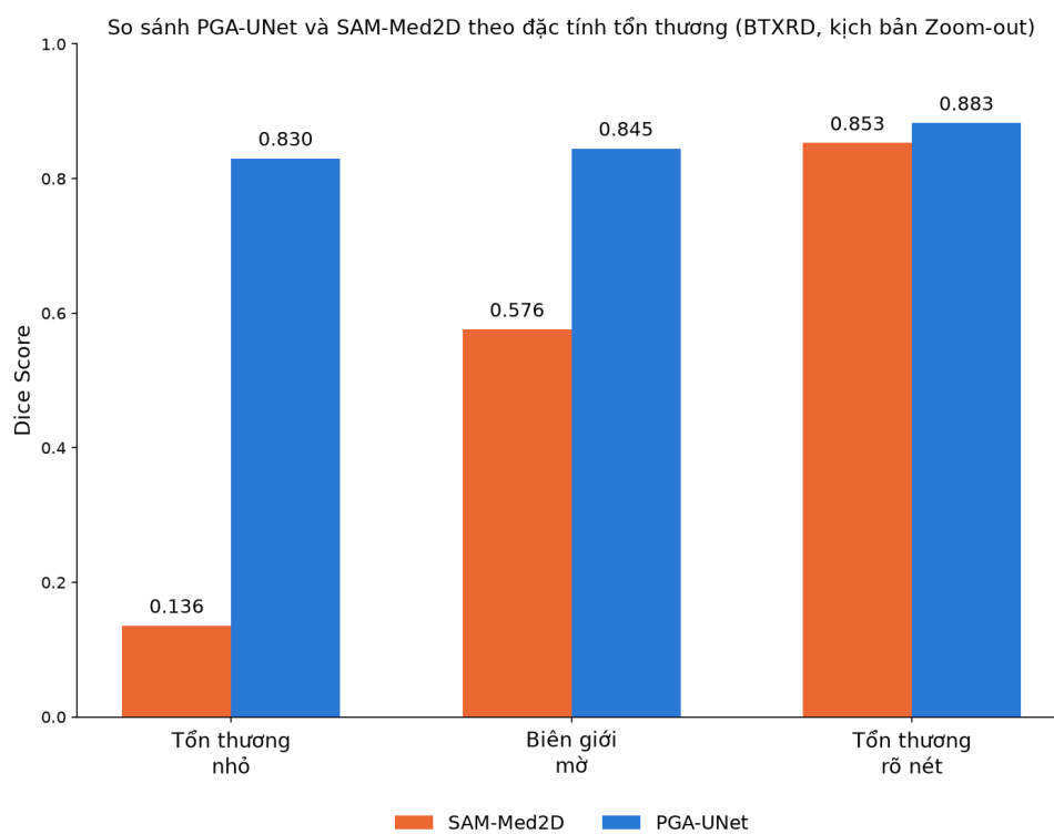
Hình 4.10: So sánh PGA-UNet và SAM-Med2D theo ba nhóm đặc tính lâm sàng trên BTXRD (Bảng 4.15).
