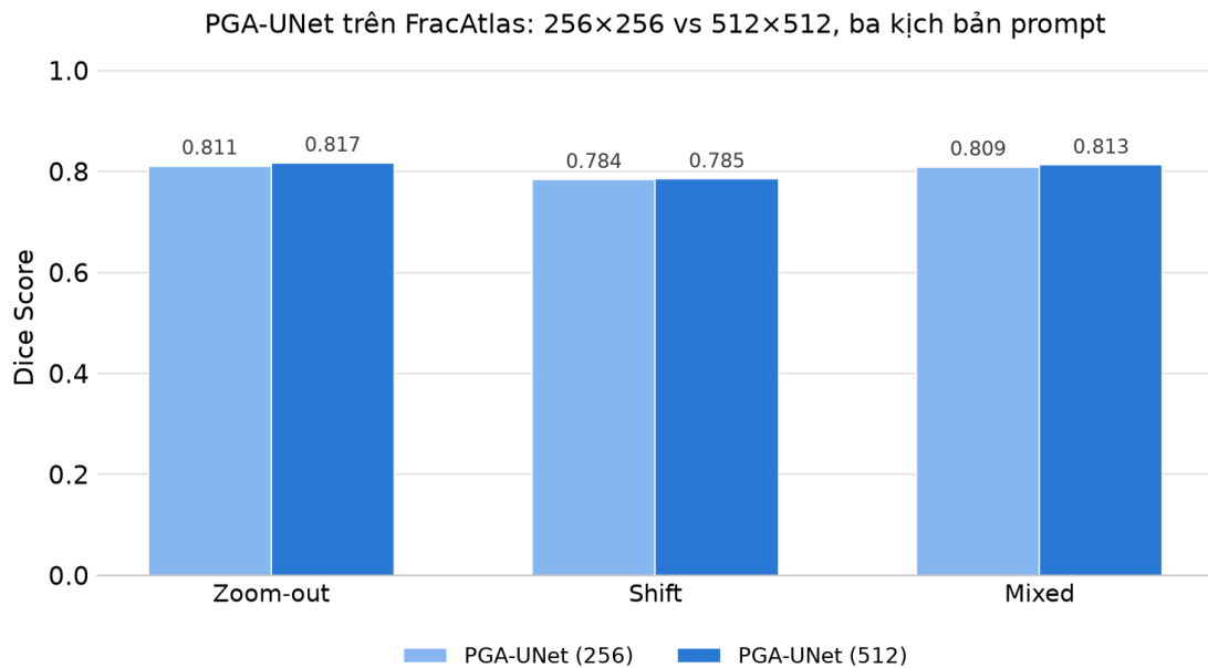
Hình 4.5: PGA-UNet trên FracAtlas: Dice Score tại 256×256 và 512×512, ba kịch bản câu nhắc (Bảng 4.9).
