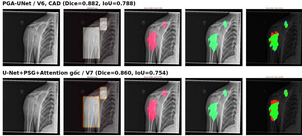
Hình 4.7: PGA-UNet/V6 (CAD) so với U-Net+PSG+Attention gốc/V7 trên cùng một ca, BTXRD, kịch bản Zoom-out.
