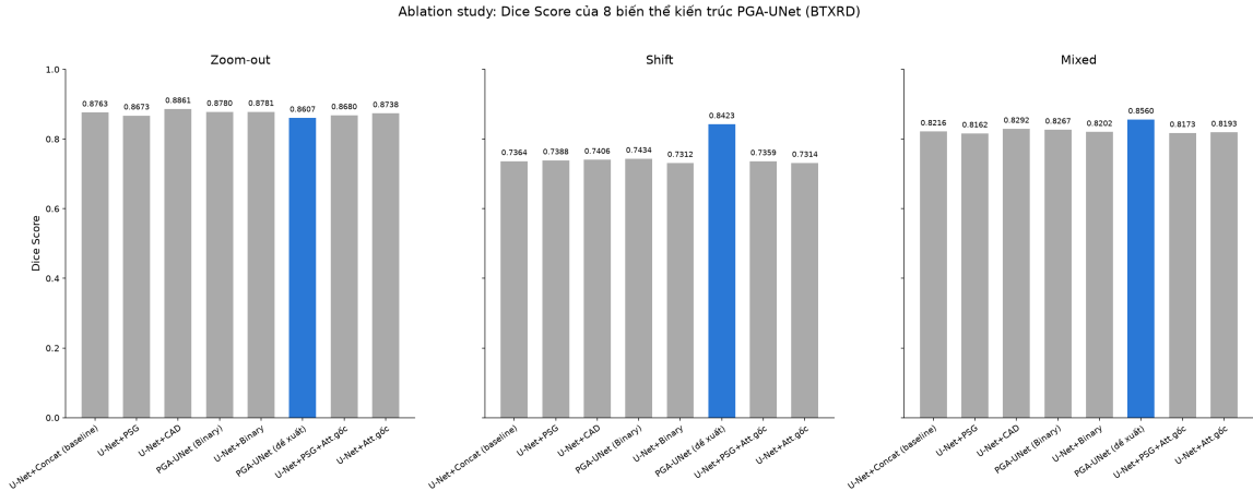
Hình 4.6: Ablation study: Dice Score của 8 biến thể kiến trúc PGA-UNet trên ba kịch bản câu nhắc (Bảng 4.11). PGA-UNet (đề xuất) tô xanh dương, các biến thể còn lại tô xám.
