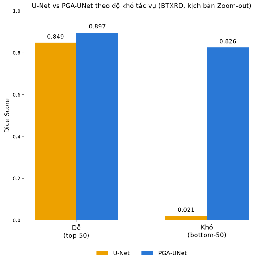
Hình 4.8: So sánh U-Net và PGA-UNet theo độ khó tác vụ trên BTXRD (Bảng 4.14).
