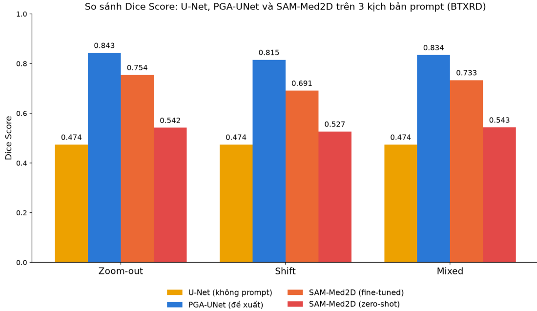
Hình 4.3: Dice Score: U-Net ( 512 \times 512 ), PGA-UNet ( 256 \times 256 ), SAM-Med2D (đã/chưa tinh chỉnh, 256 \times 256 ), ba kịch bản câu nhắc trên BTXRD (Bảng 4.3, 4.6).
