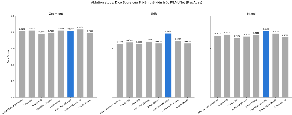
Hình 4.12: Ablation study: Dice Score của 8 biến thể kiến trúc PGA-UNet trên ba kịch bản câu nhắc trên FracAtlas (Bảng 4.17). PGA-UNet (đề xuất) tô xanh dương, các biến thể còn lại tô xám.
