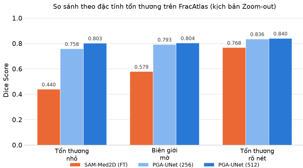
Hình 4.16: So sánh SAM-Med2D (FT), PGA-UNet (256) và PGA-UNet (512) theo ba nhóm đặc tính tổn thương trên FracAtlas (Bảng 4.21).
