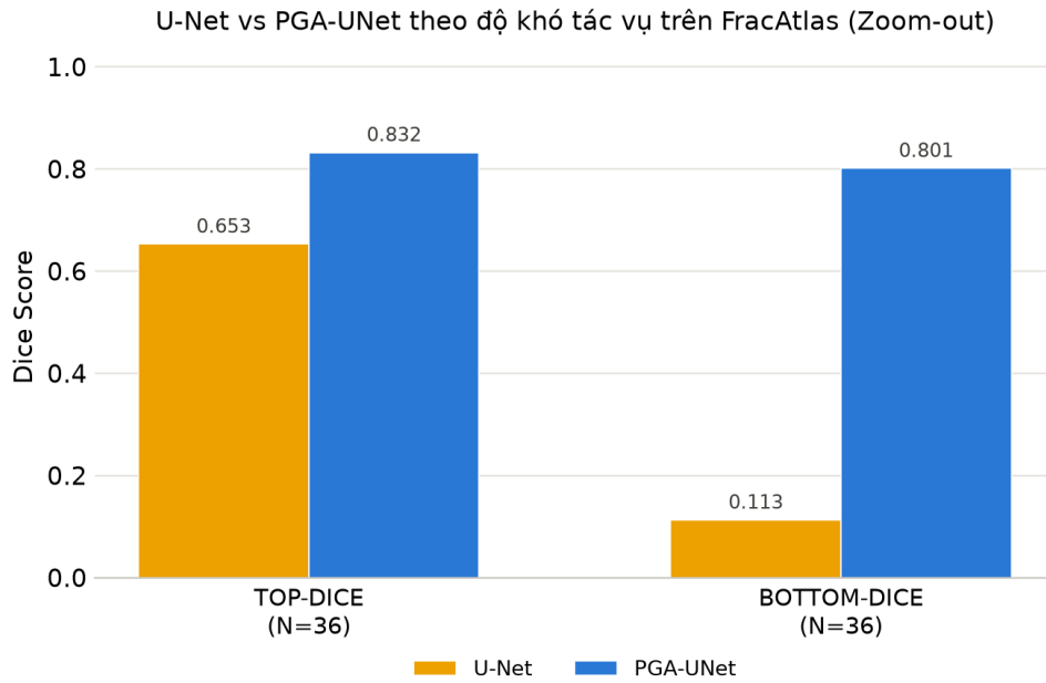
Hình 4.14: So sánh U-Net và PGA-UNet theo độ khó tác vụ trên FracAtlas (Bảng 4.20).
