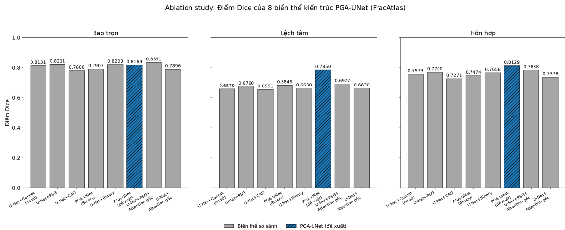
Hình 4.10: Dice của tám cấu hình trong nghiên cứu loại bỏ thành phần trên FracAtlas. PGA-UNet đề xuất đạt kết quả cao nhất trong hai kịch bản Lệnh tâm và Hỗn hợp.
