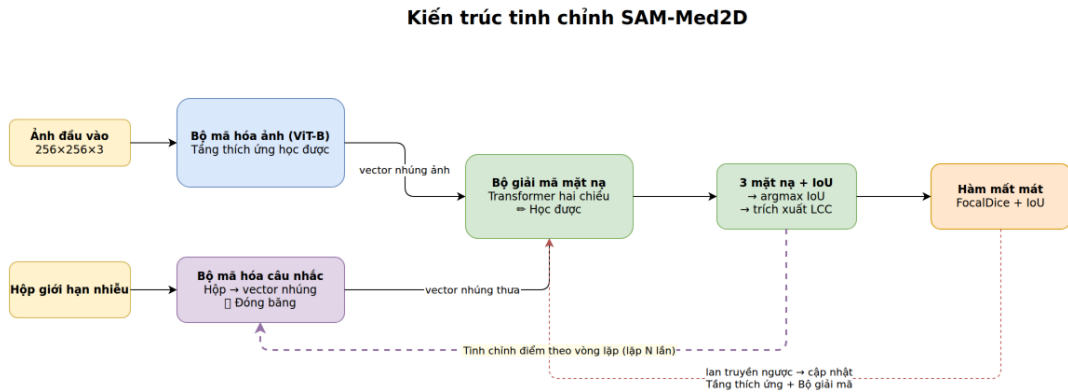
Hình 2.1: Kiến trúc tổng quát của SAM-Med2D [3].
