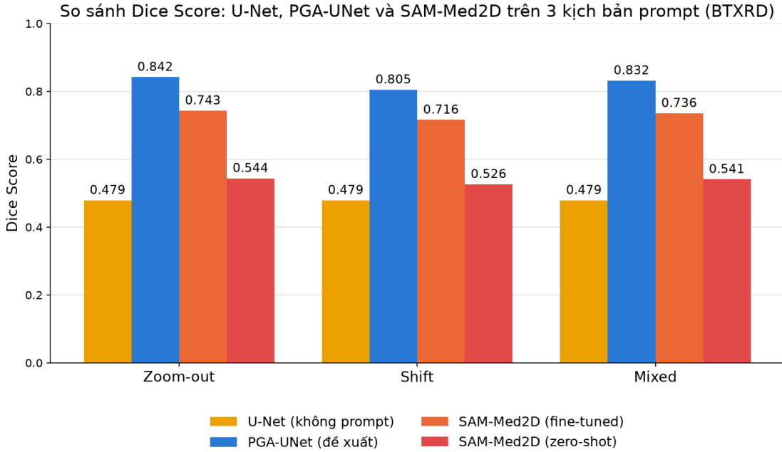
Hình 4.1: So sánh Dice Score giữa U-Net (không prompt, 512 \times 512 ), PGA-UNet ( 256 \times 256 ) và SAM-Med2D (fine-tuned, zero-shot, 256 \times 256 ) trên ba kịch bản prompt, tổng hợp trực quan từ Bảng 4.2 và 4.4.
