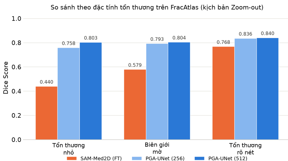
Hình 4.6: So sánh SAM-Med2D (FT), PGA-UNet (256) và PGA-UNet (512) theo ba nhóm đặc tính tổn thương trên FracAtlas (Bảng 4.17).
