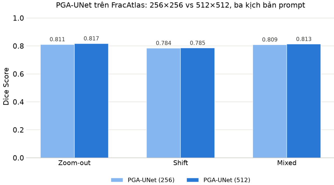
Hình 4.4: PGA-UNet trên FracAtlas: Dice Score tại 256 \times 256 và 512 \times 512 , ba kịch bản prompt (Bảng 4.13).
