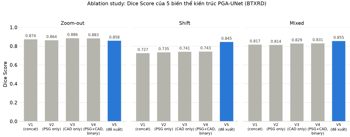
Hình 4.2: Ablation study: Dice Score của 5 biến thể kiến trúc PGA-UNet trên ba kịch bản prompt (Bảng 4.6). V5 (đề xuất, xanh dương) thấp hơn nhẹ ở Zoom-out nhưng vượt trội rõ rệt ở Shift so với bốn biến thể còn lại (xám).
