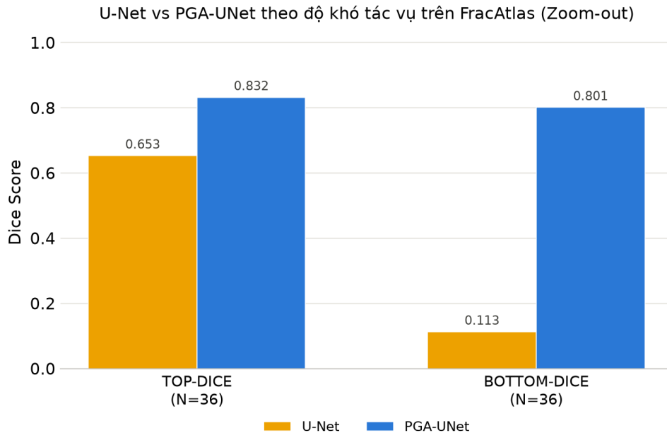
Hình 4.5: So sánh U-Net và PGA-UNet theo độ khó tác vụ trên FracAtlas (Bảng 4.16).
