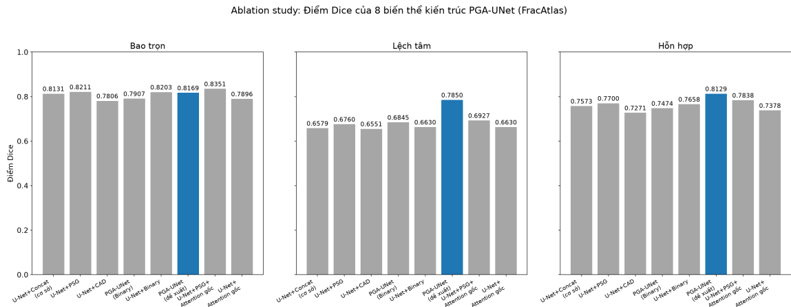
Hình 4.11: Nghiên cứu loại bỏ thành phần: Điểm Dice của 8 biến thể kiến trúc PGA-UNet trên ba kịch bản câu nhắc trên FracAtlas (Bảng 4.16). PGA-UNet (đề xuất) tô xanh dương, các biến thể còn lại tô xám.
