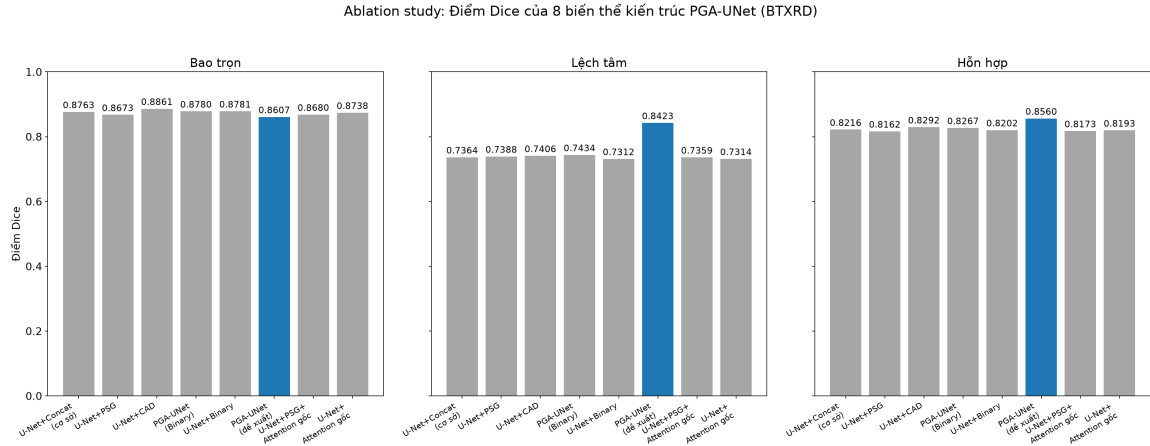
Hình 4.5: Nghiên cứu loại bỏ thành phần: Điểm Dice của 8 biến thể kiến trúc PGA-UNet trên ba kịch bản câu nhắc (Bảng 4.10). PGA-UNet (đề xuất) tô xanh dương, các biến thể còn lại tô xám.
