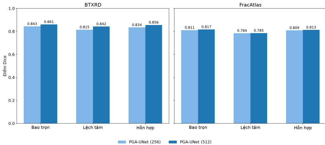
Hình 4.3: PGA-UNet tại 256 \times 256 và 512 \times 512 , ba kịch bản câu nhắc: BTXRD so với FracAtlas (Bảng 4.7, 4.8).
