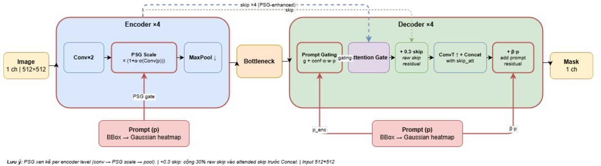
Hình 3.3: Kiến trúc PGA-UNet (Prompt-Guided Attention U-Net): Cổng không gian (Prompt Spatial Gate) tích hợp bản đồ nhiệt câu nhắc vào bộ mã hóa để tăng cường đặc trưng có chọn lọc; Cơ chế chú ý có điều kiện (Conditioned Attention) ràng buộc tín hiệu gating bằng câu nhắc tại từng tầng giải mã với trọng số giảm dần
