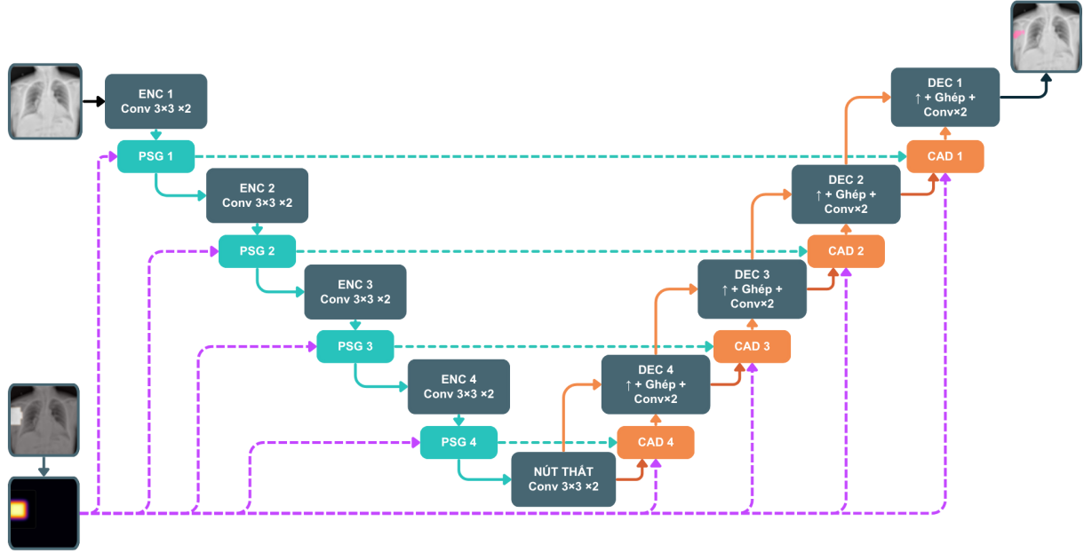
Hình 3.1: Kiến trúc PGA-UNet với PSG tại bộ mã hóa và CAD tại bộ giải mã.
