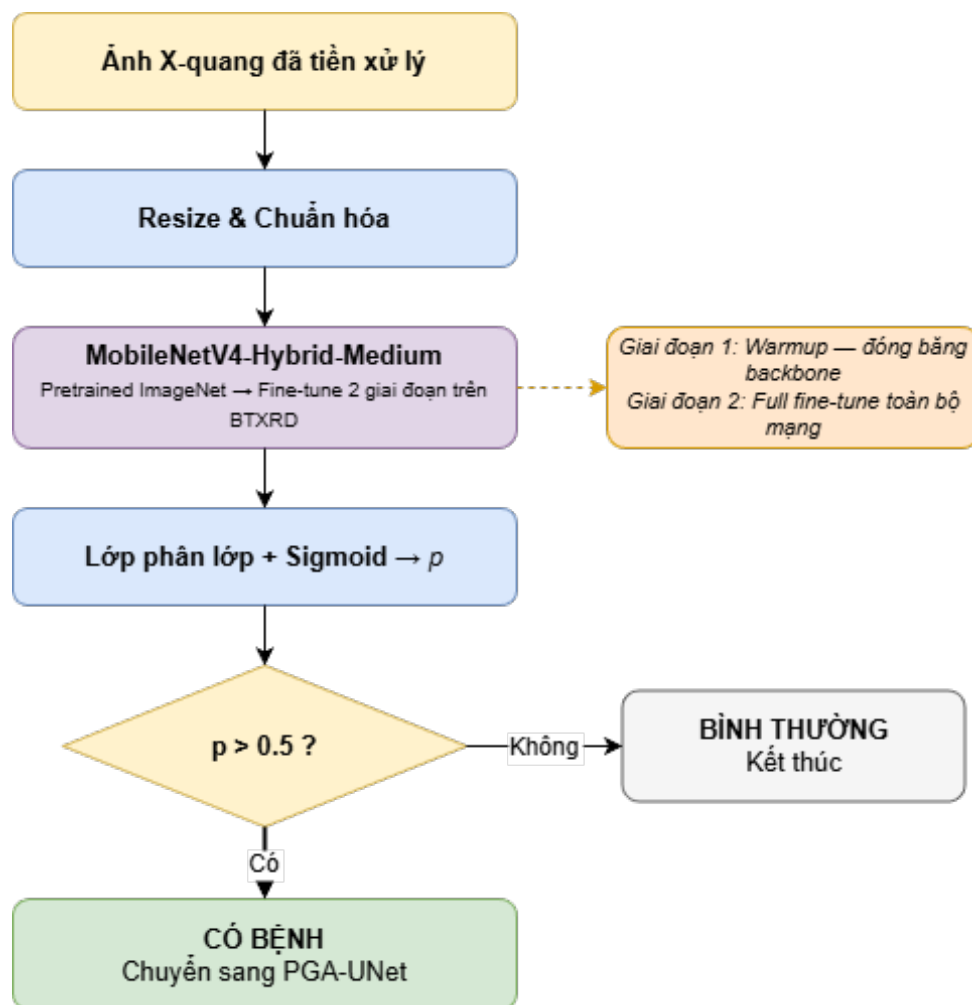
Hình 3.6: Pipeline phân lớp nhị phân MobileNetV4 Gatekeeper: resize và chuẩn hóa ảnh đầu vào, backbone MobileNetV4-Hybrid-Medium được tinh chỉnh hai giai đoạn (warmup đồng bằng → full fine-tune), lớp phân lớp tuyến tính và Sigmoid với ngưỡng 0.5 quyết định CÓ/KHÔNG bệnh lý
