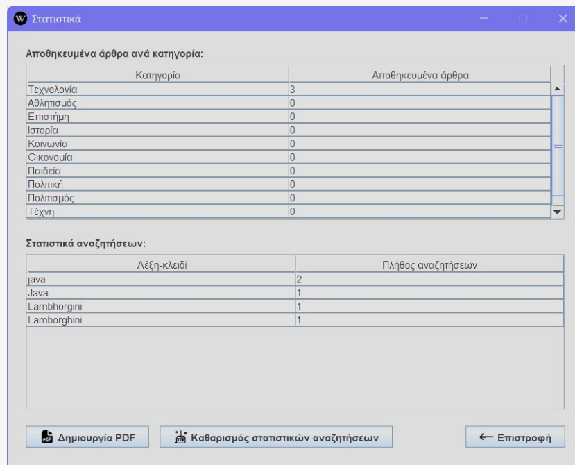
Εικόνα 9: Οθόνη Στατιστικών
