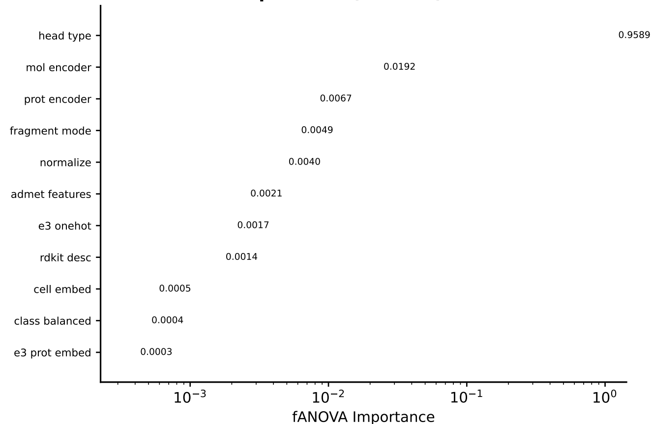
B Parameter Importance (fANOVA)
