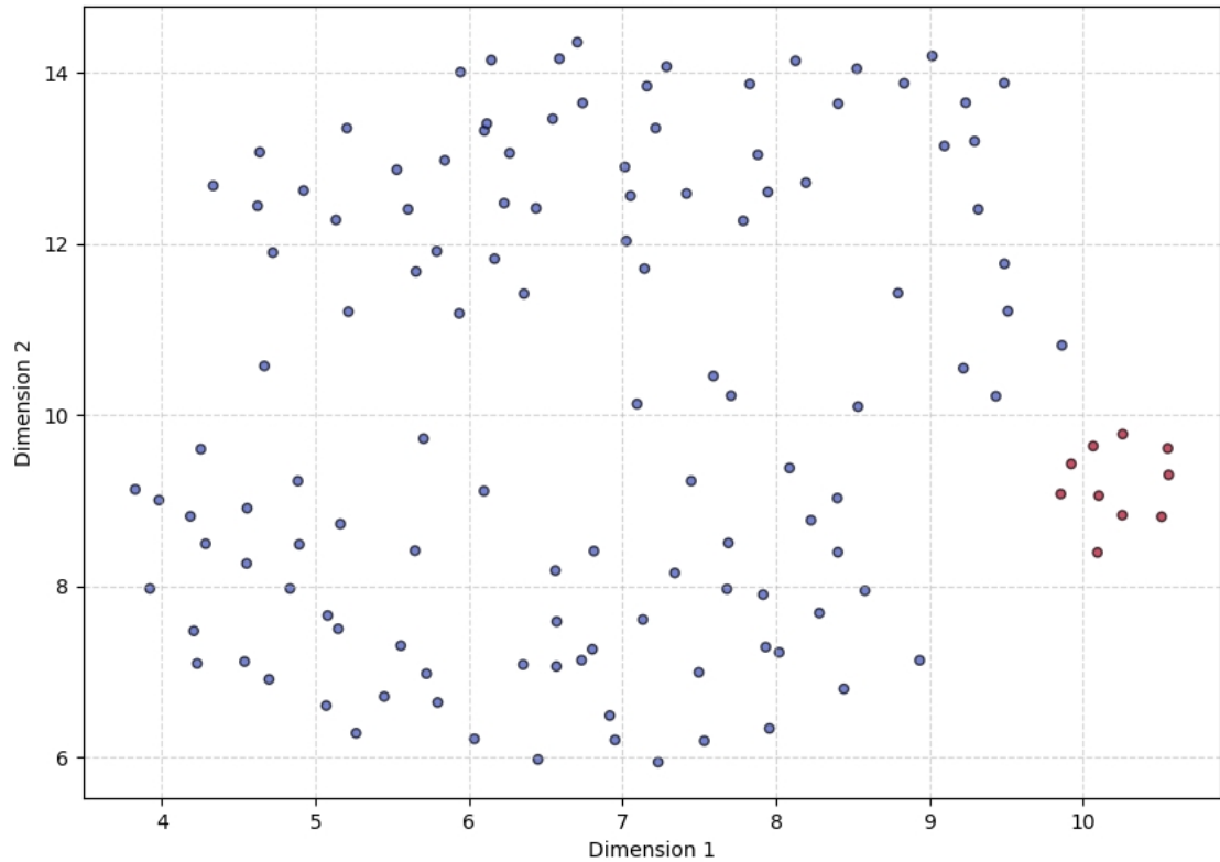
UMAP Visualization
