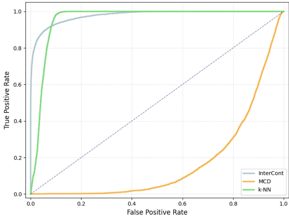
ROC-AUC
