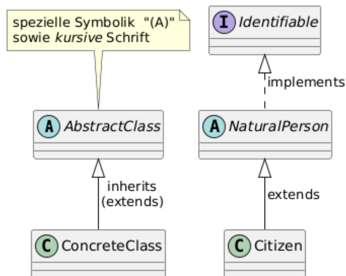
Figure 2. Abstrakte Klassen & Vererbung
