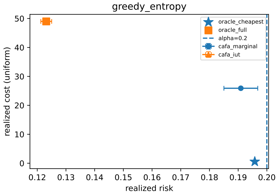
F1 realized (risk, cost) -- mnist ts1 (lambda_ref=0.9)
