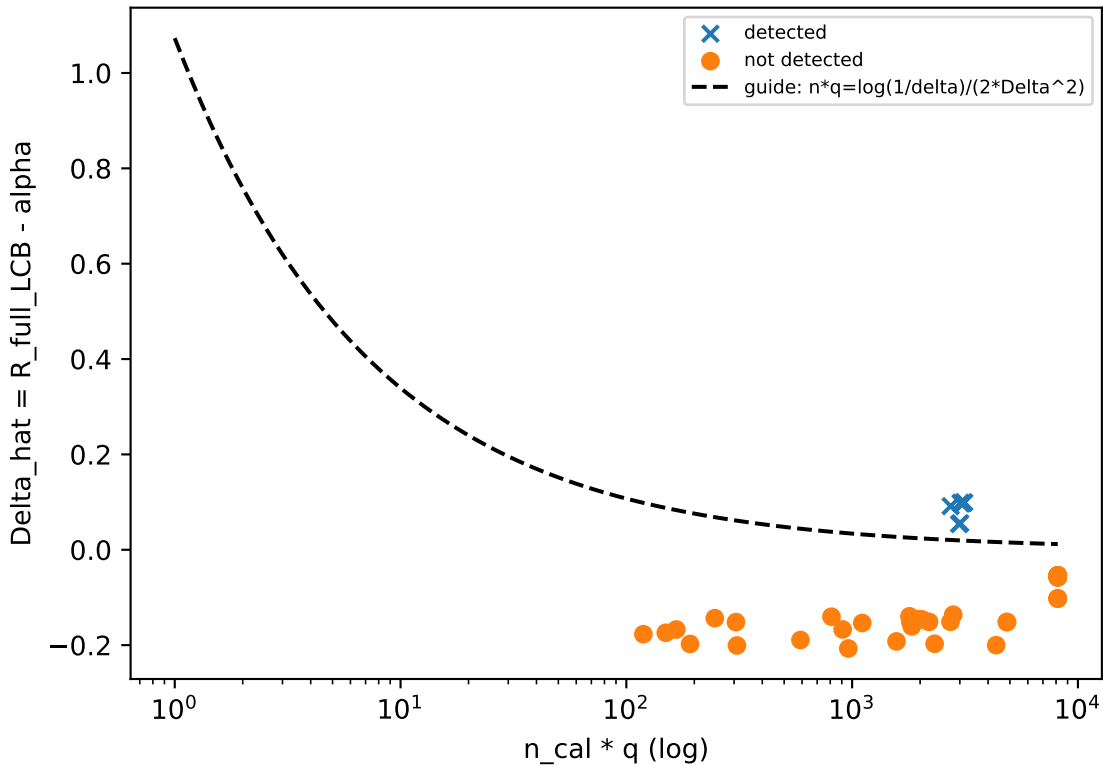
F4 detection -- tabular-adult
