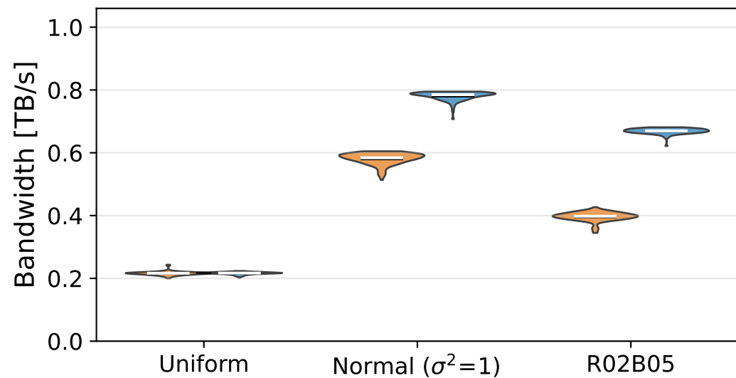
MI300A Zen Cores
