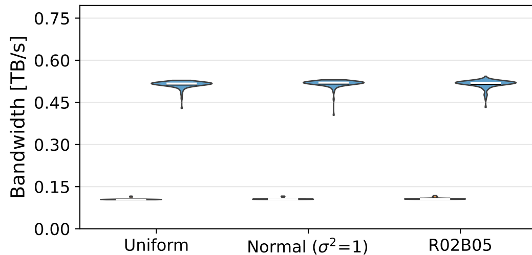
MI300A Zen Cores
