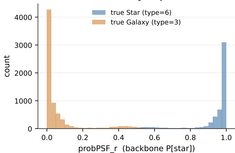
(d) Backbone star/galaxy confidence
