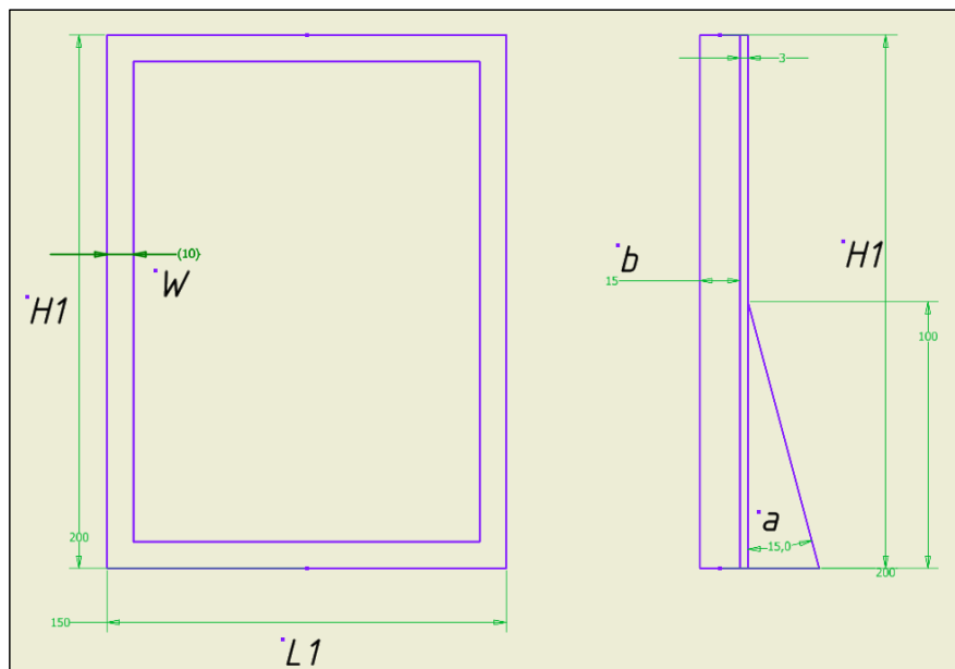
Рисунок 2.1 — Модель Рамки для фотографии с размерами
