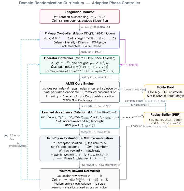
Hình 2: Kiến trúc Hierarchical MDP temporally-coupled của hệ thống Hybrid DDQN-ALNS, kết hợp Plateau Controller, Operator Controller, ALNS Core Engine, LAC và Welford Normalizer trong một vòng lặp học-tối ưu. Ký hiệu luồng: Mũi tên liền nét (luồng dữ liệu tiến), Mũi tên đứt nét màu xanh (vòng phản hồi phần thưởng), Mũi tên màu hồng/magenta (vector chế độ điều phối mục tiêu).
