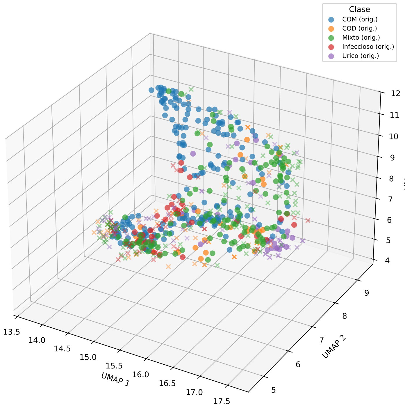
Originales (•) vs aumentadas (x) en el espacio LBP+HSV (3D)
