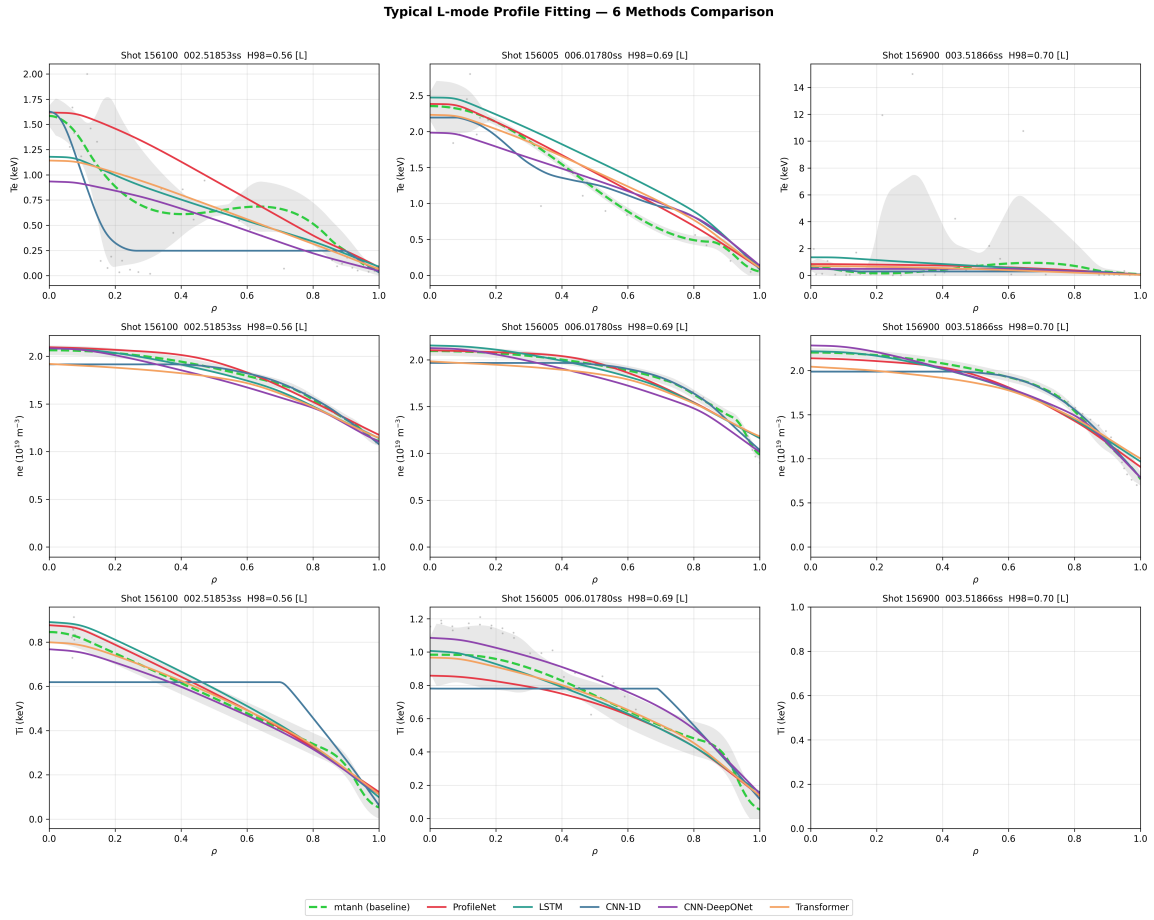
图 5: 典型 L 模剖面拟合结果: 六种方法在三个代表性 L 模时间点上对 T_e 、 n_e 、 T_i 三种诊断的对比, 验收区间阴影与图 2 同口径。
