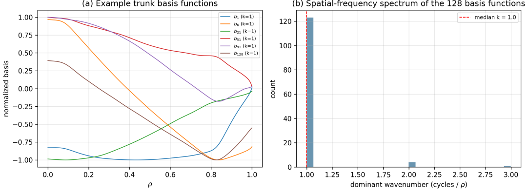
图 8: 共享 CoordDecoder 的空间频率内容: (a) 六个示例主干基函数 b_k(\rho) ; (b) 全部 128 个基函数主导波数 (FFT 峰值) 的直方图。所有基函数的主导波数均 \leq 3 周期/单位 \rho (中位数 1), 定量刻画了 DeepONet 输出空间的结构性光滑。
