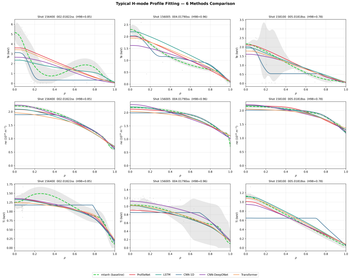
图 2: 典型 H 模剖面拟合结果: 六种方法 (mtanh 基线 + 五种 NN 架构) 在三个代表性 H 模时间点上对 T_e 、 n_e 、 T_i 三种诊断的对比。灰色阴影带为数据驱动验收区间, 定义见第 3 节。所示时间点为测试集各 H 模炮中最接近 H 模 H_{98} 中位数的点 (此处 0.78–0.96, 每炮一个), 并经过第 3 节所述自动质量筛查。
