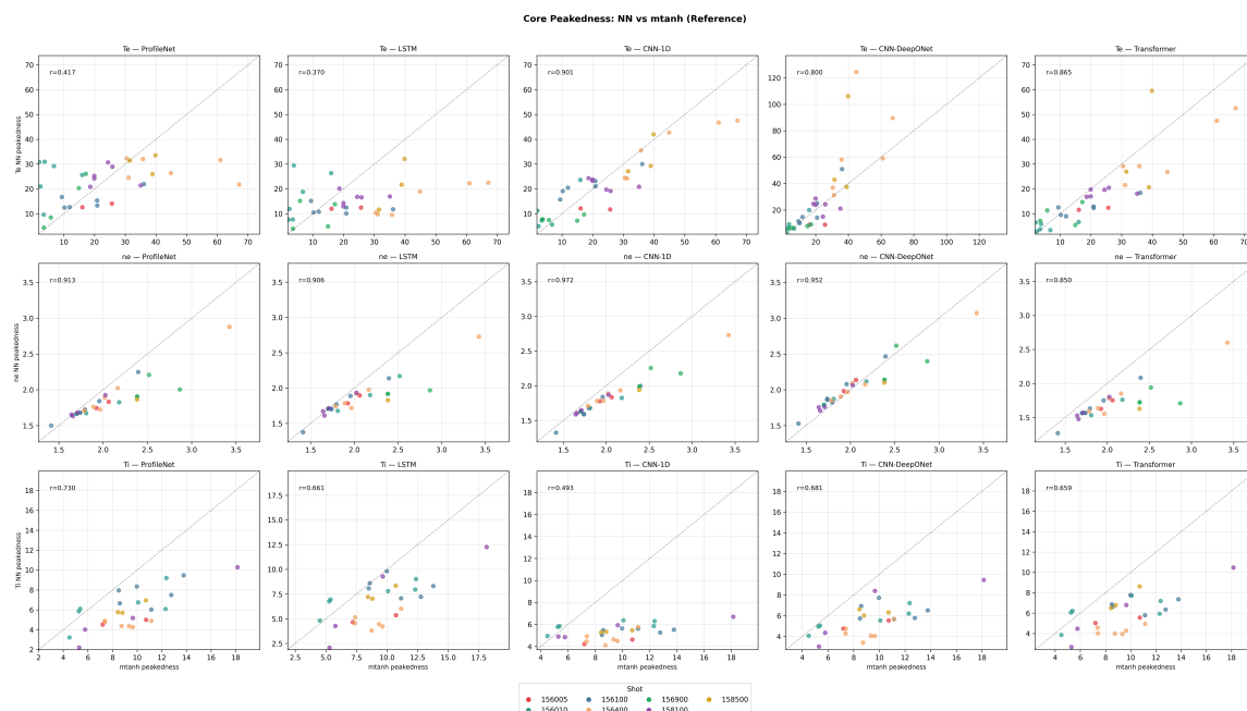
图 7: 芯部峰值度 ( y_{core}/y_{edge} ): NN 预测值 vs. mtanh 参考值。每个点代表一个时间点, 颜色按炮号区分。对角线虚线表示完全一致; 图中标注了 Pearson r 值。
